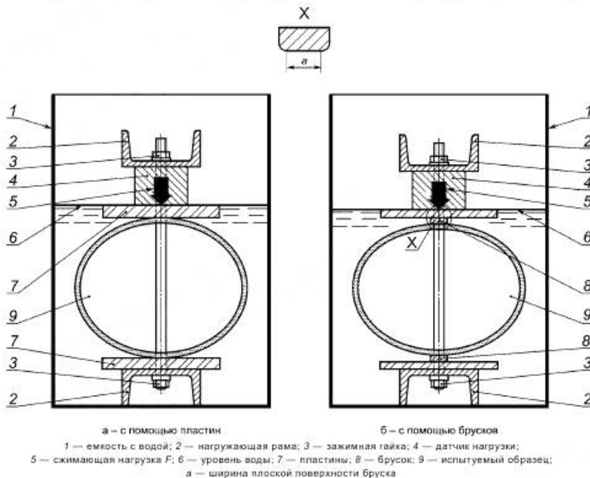
Рисунок 1 — Схемы нагружения образца
