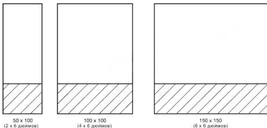
Рисунок Х1.2 — Размеры образцов
