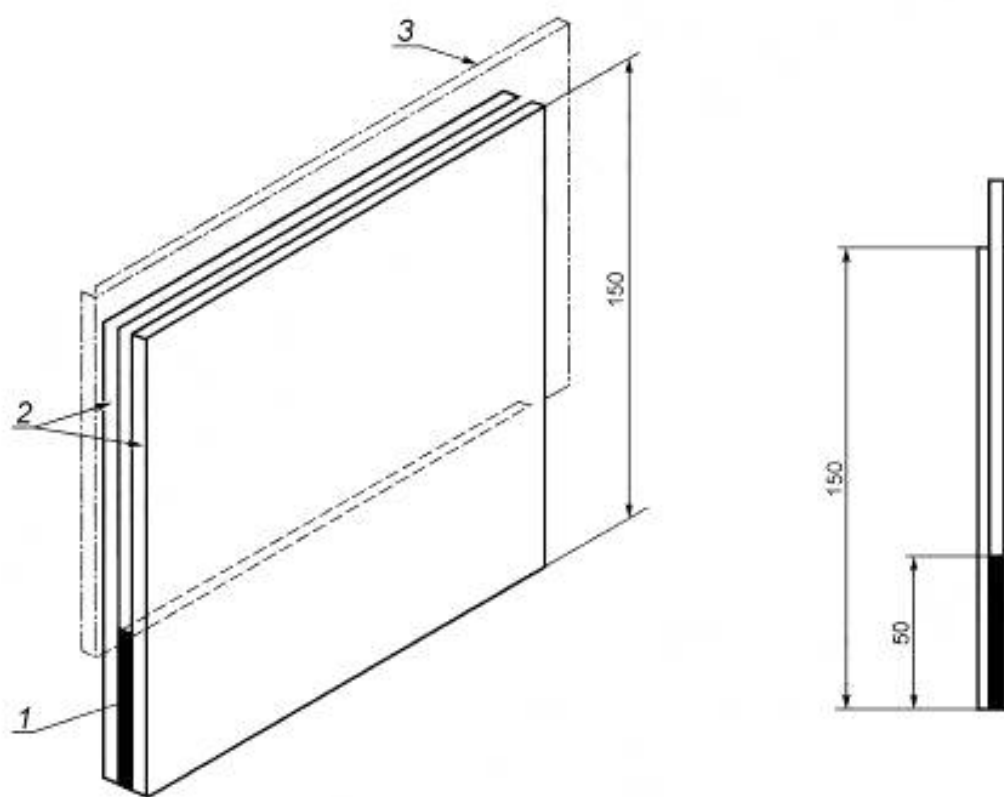
Рисунок 5 — Образец для испытания в сборе
