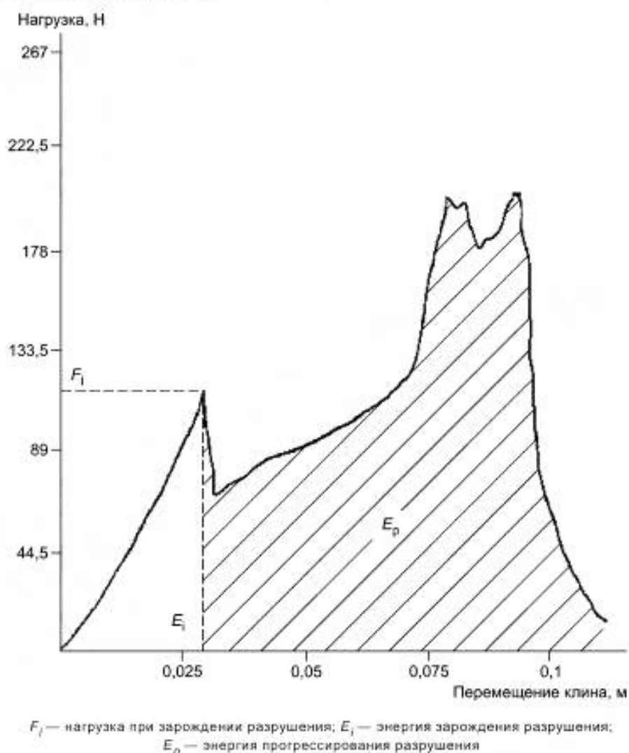
Рисунок 1 — График зависимости изменения нагрузки от перемещения клина
