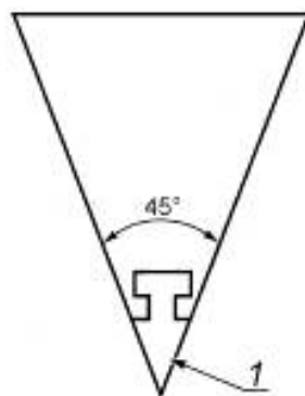
1 — съёмный наконечник
