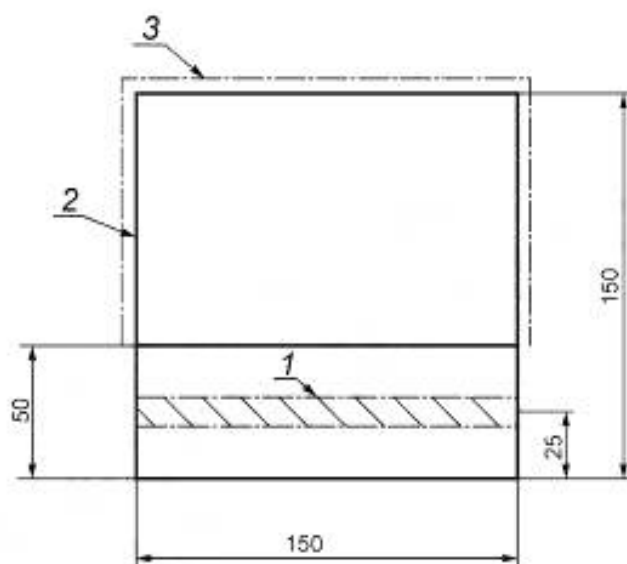
1 — клеевой шов; 2 — подложка; 3 — съемная прокладка
