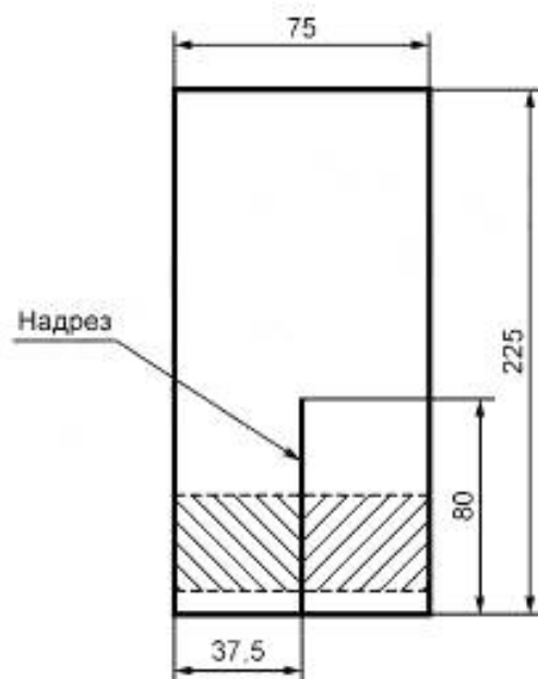
Рисунок 2 — Образец с двумя язычками
