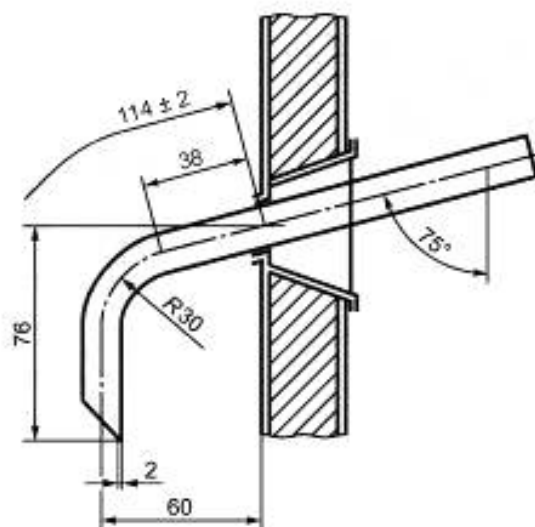
Рисунок А2.3 — Нижний конец трубки холодильника
