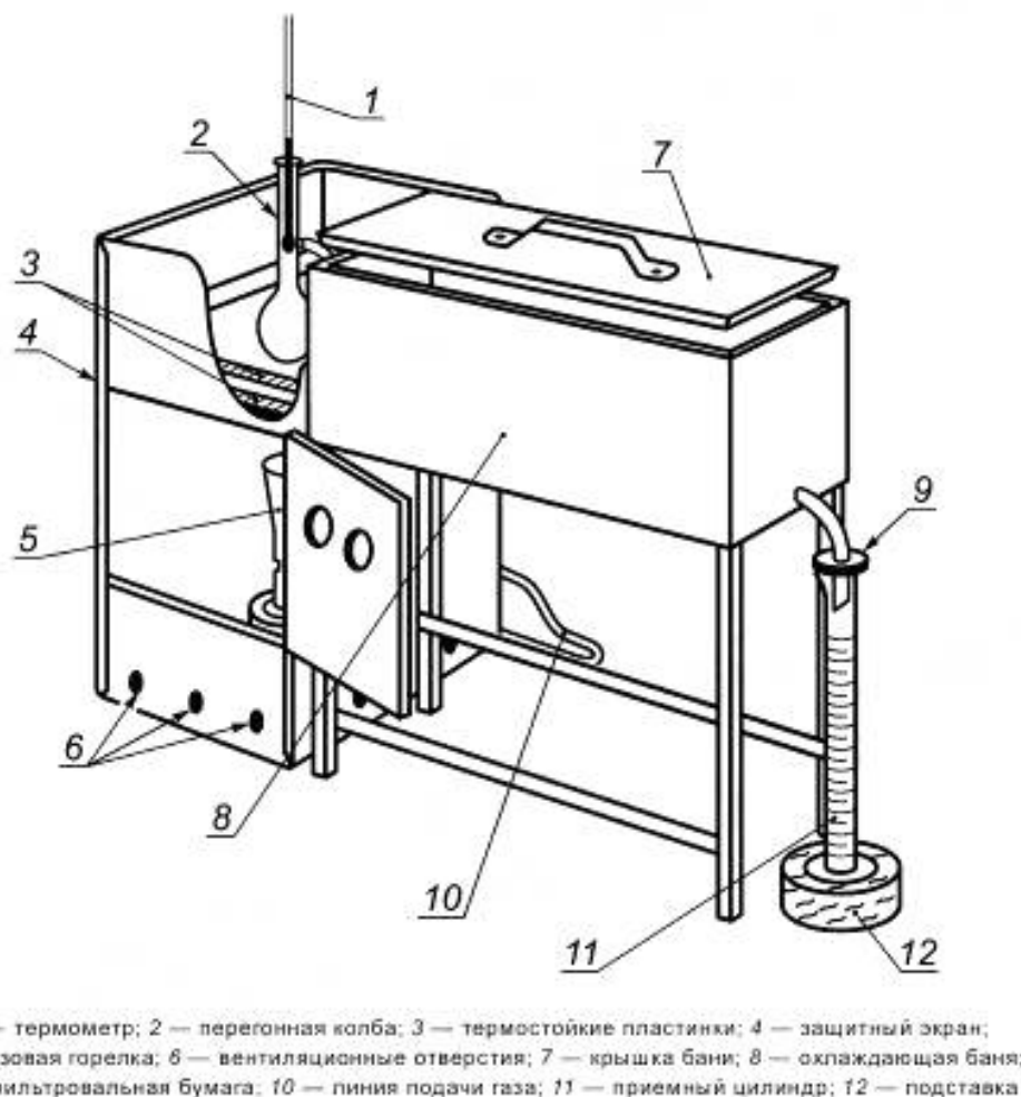
Рисунок 1 — Аппарат в сборе с газовой горелкой
