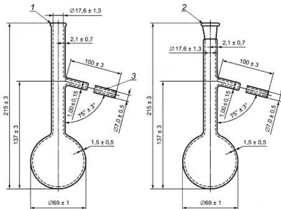
1 — усиливающий валик; 2 — муфта 19/22 или 19/26; 3 — огневая полировка стекла
