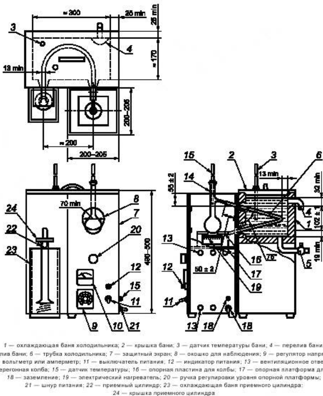
Рисунок 2 — Аппарат в сборе с электрическим нагревателем
