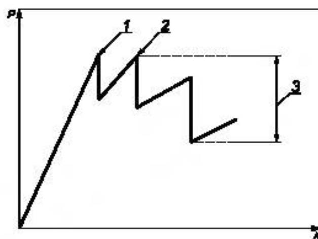
Рисунок 3 — Типовая зависимость P/\Delta для однонаправленного образца
