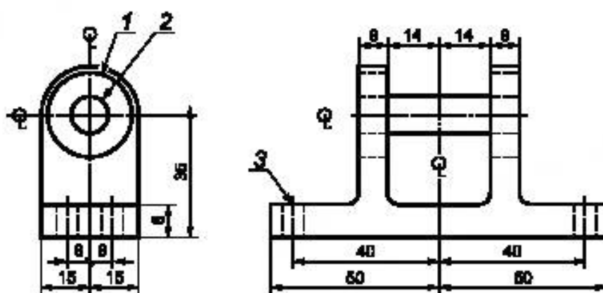
1 — подшипник, установленный в опору; 2 — отверстие под штангу, 10 мм; 3 — отверстие 5 мм (в 4 местах) б — Нижнее несущее крепление (необходимо 2 шт.)
