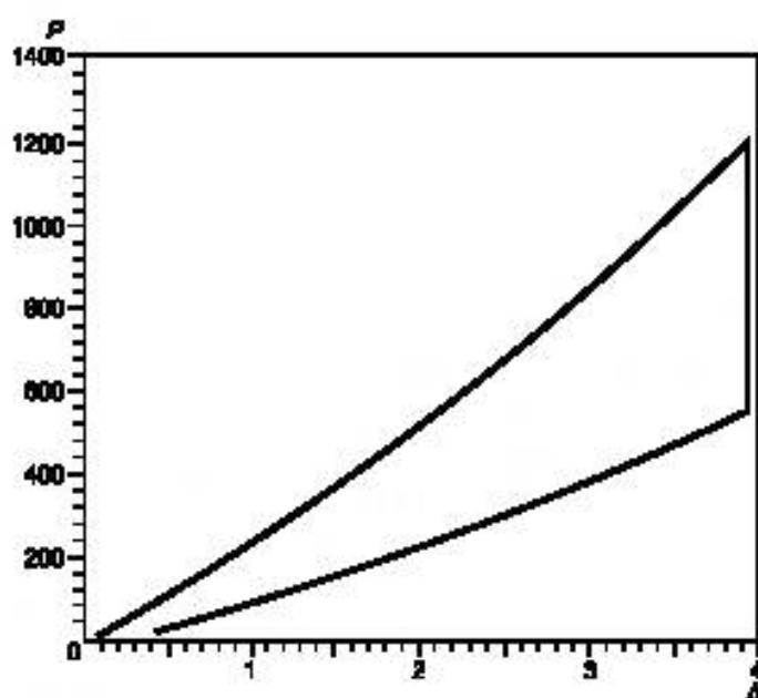
Рисунок 3 — Типовая зависимость P/\Delta для однонаправленного образца
