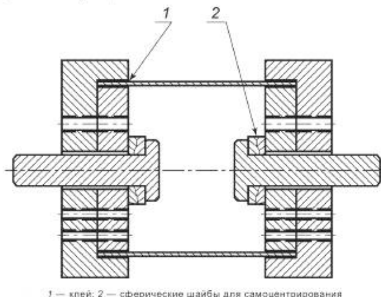
1 — клей; 2 — сферические шайбы для самоцентрирования
