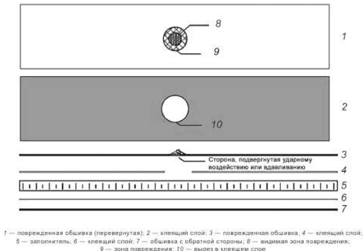
Рисунок 1 — Изготовление «сэндвич»-конструкции
