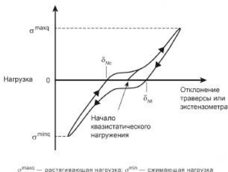
Рисунок 2 — Параметры петли гистерезиса для расчета смещения крепежа в зависимости от количества циклов нагружения
