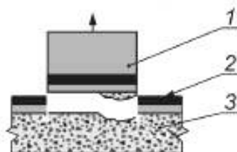
Рисунок В.5 — Отрыв типа Д (отрыв по границе соединения адгезионного слоя и бетонного основания)
