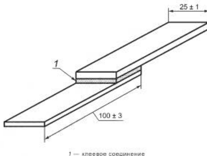
Рисунок 1 — Соединение внахлест
