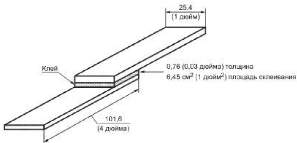
Рисунок 1 — Соединение внахлест
