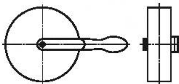
Рисунок 1 — Валик для прикатки образцов
