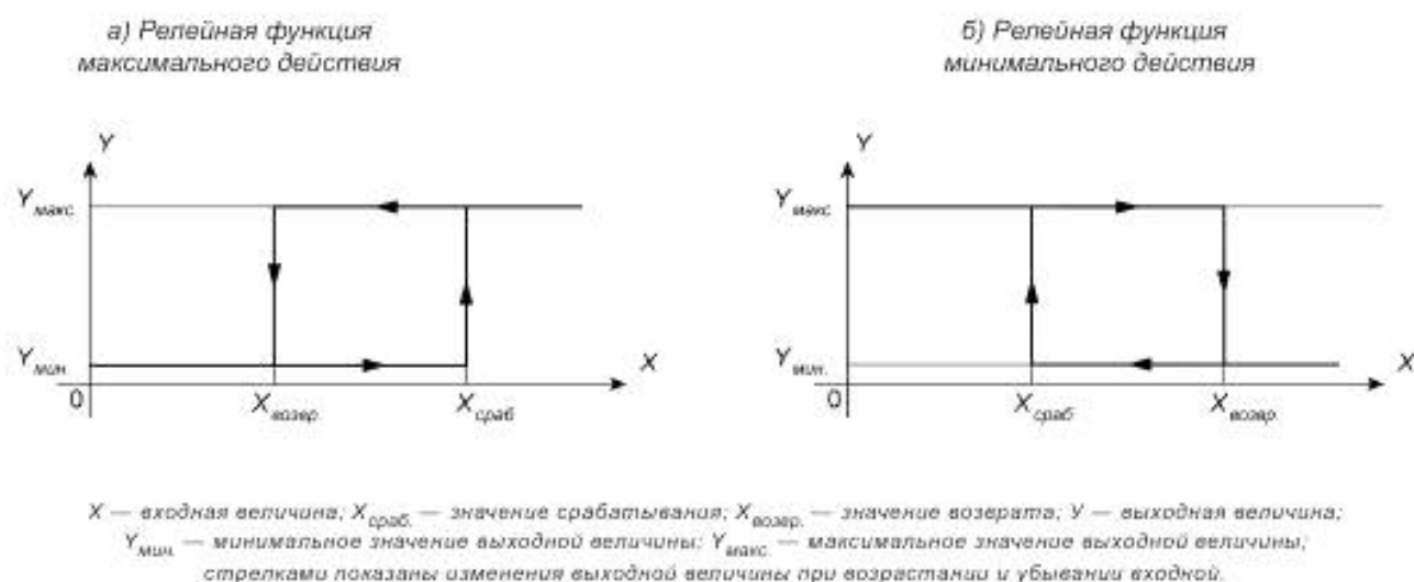
Рисунок 1 — Графики релейных функций одной входной величины
