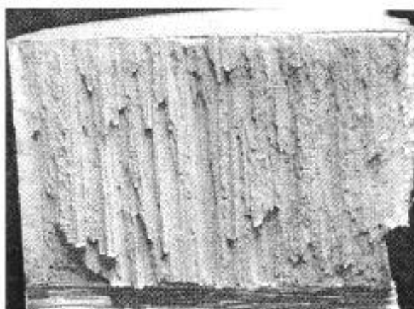
Излом
