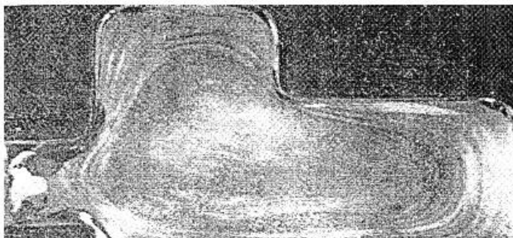
Макроструктура профиля
