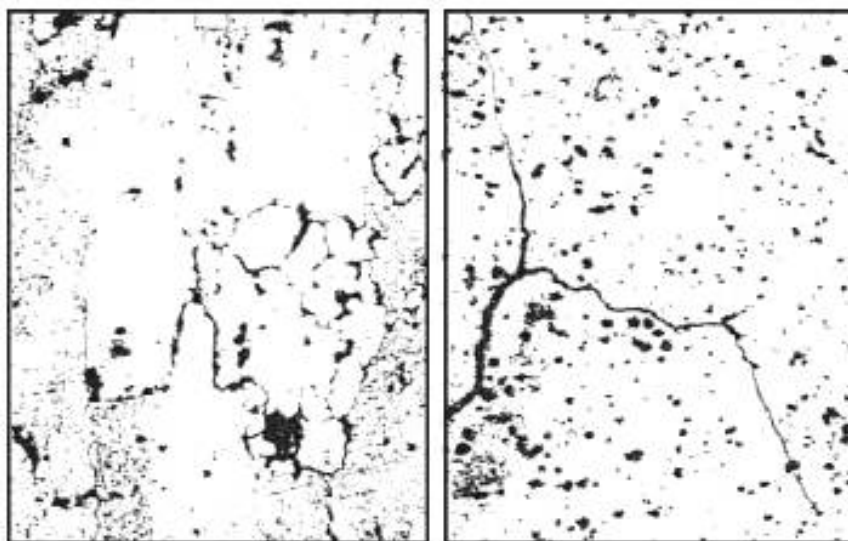
Микроструктура пережога × 300
