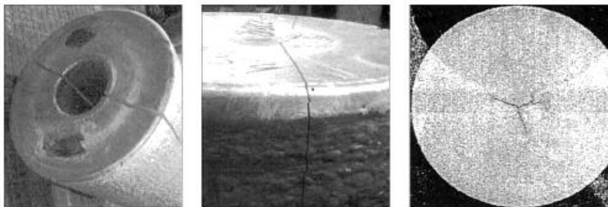
Рисунок А.6 — Трещина центральная
