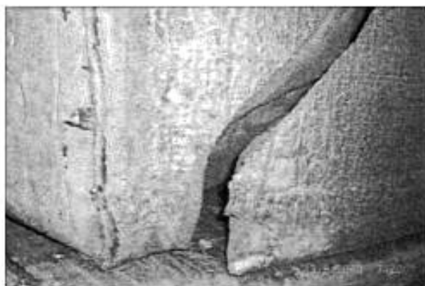
Рисунок А.7 — Трещина боковая
