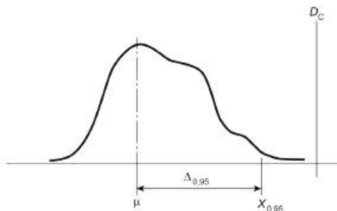
Рисунок Б.1 — График для определения величин X_{0,95} и \Delta_{0,95}
