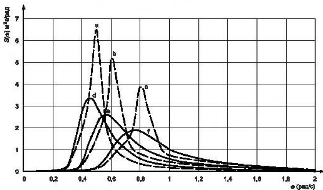
Рисунок Б.1 — Спектры Пирсона-Московица и JONSWAP — H_s = 4,0 м, равные пиковые периоды: T_p = 6 с, 8 с, 10 с
