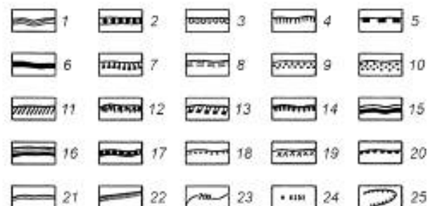
Рисунок В.8 — Типы берегов и рельеф дна Азовского моря
