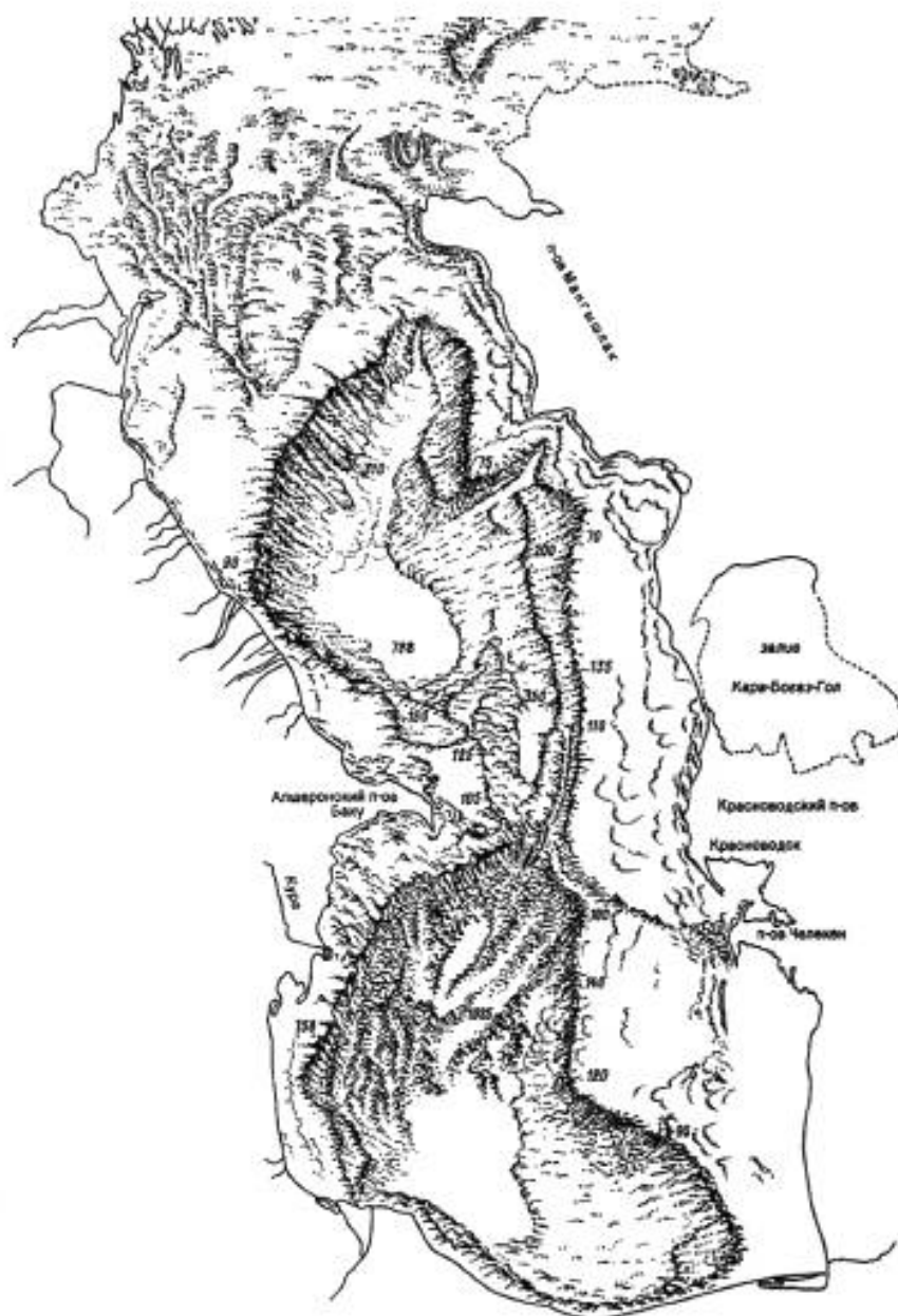
Рисунок В.2 — Физиографическая карта Каспийского моря
