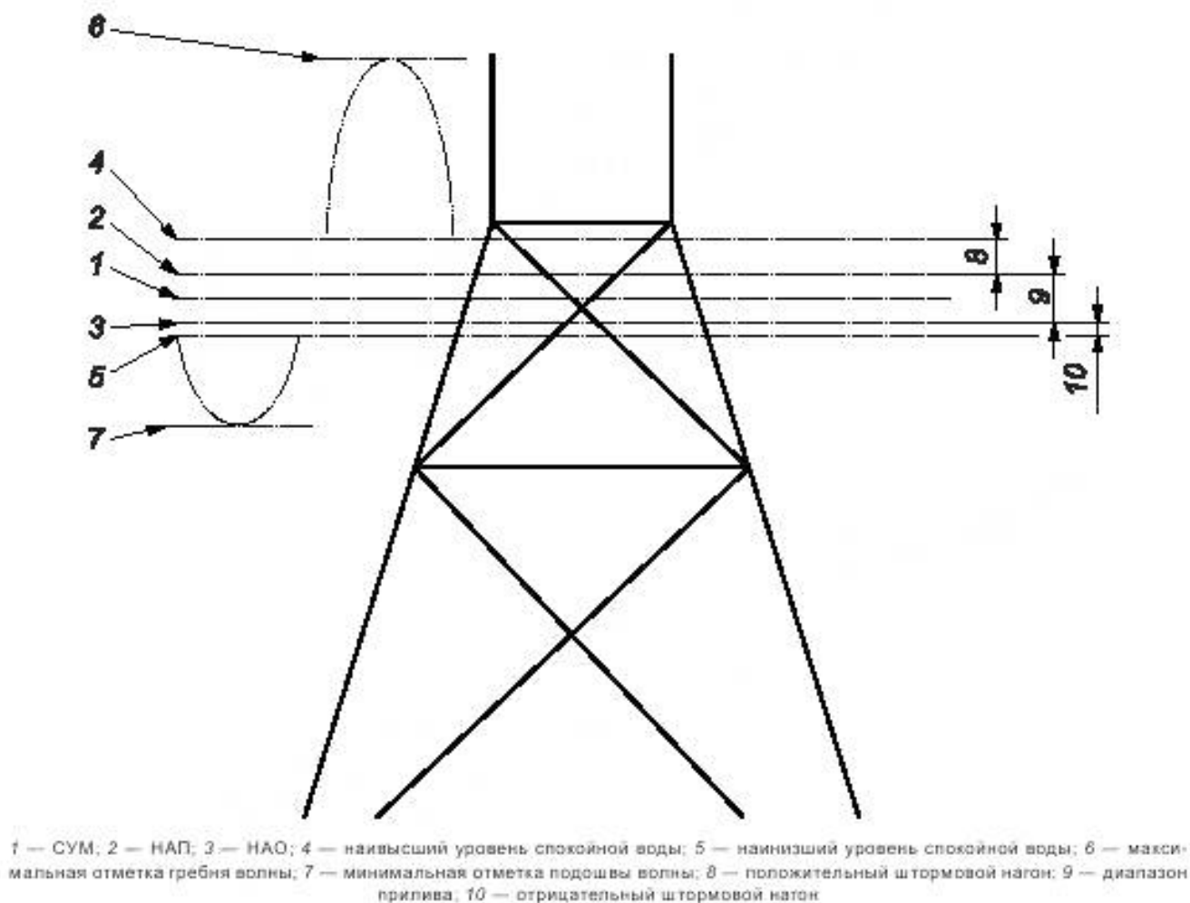
Рисунок 1 — Глубина воды, приливы и штормовые нагоны
