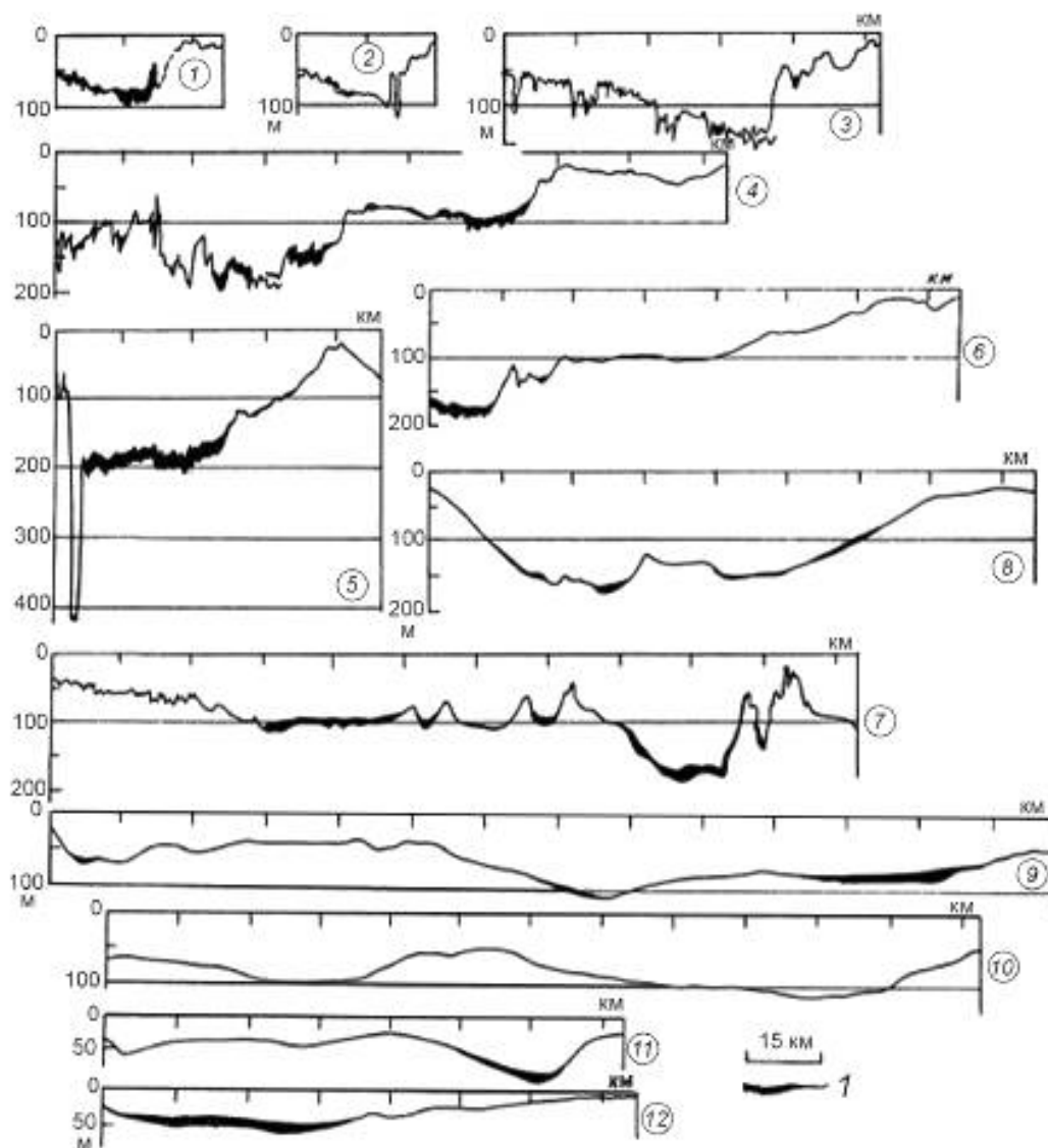
б) Профили рельефа дна Балтийского моря
