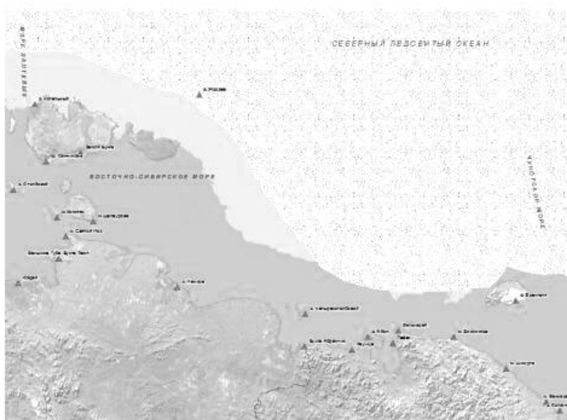
Рисунок В.24 — Схемы расположения морских гидрометстанций и постов Восточно-Сибирского моря
