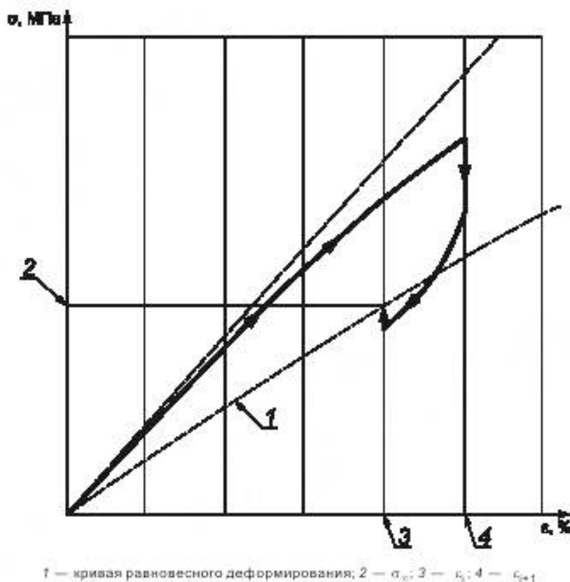
Рисунок 1 — Схема эксперимента по определению равновесного значения напряжения \sigma_v при заданной деформации \varepsilon_v
