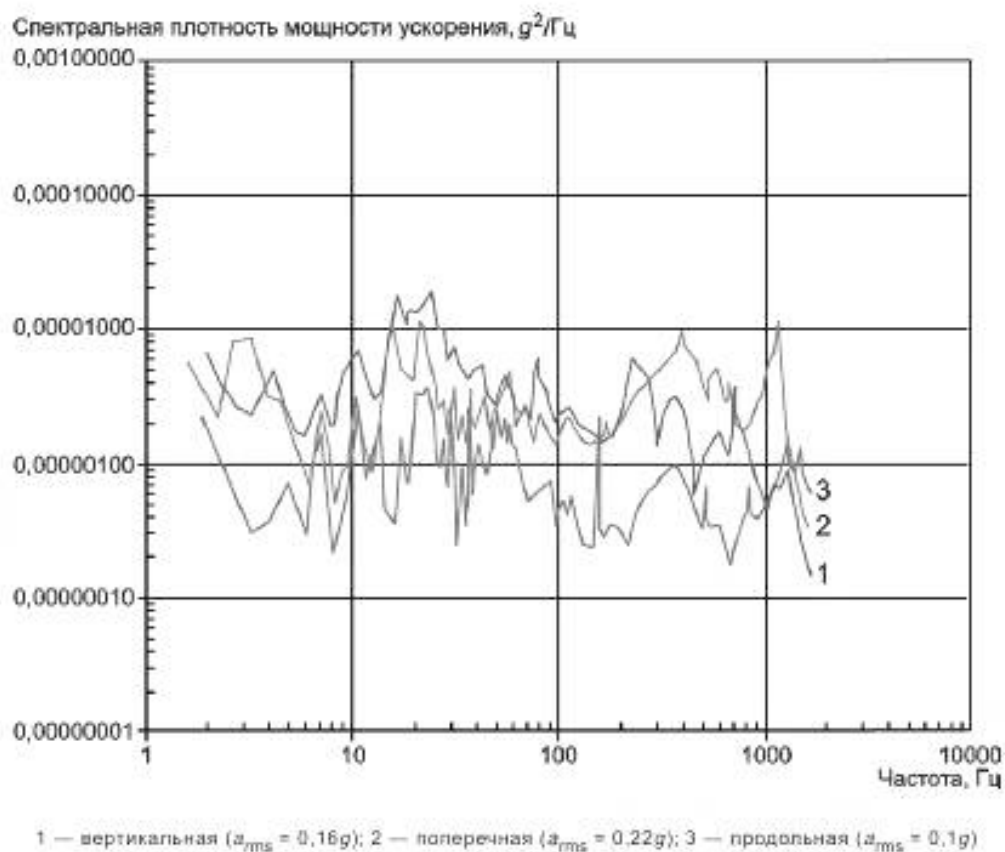
Рисунок 24 — Измерения вибрации на самолете DC8 (реверсное торможение)
