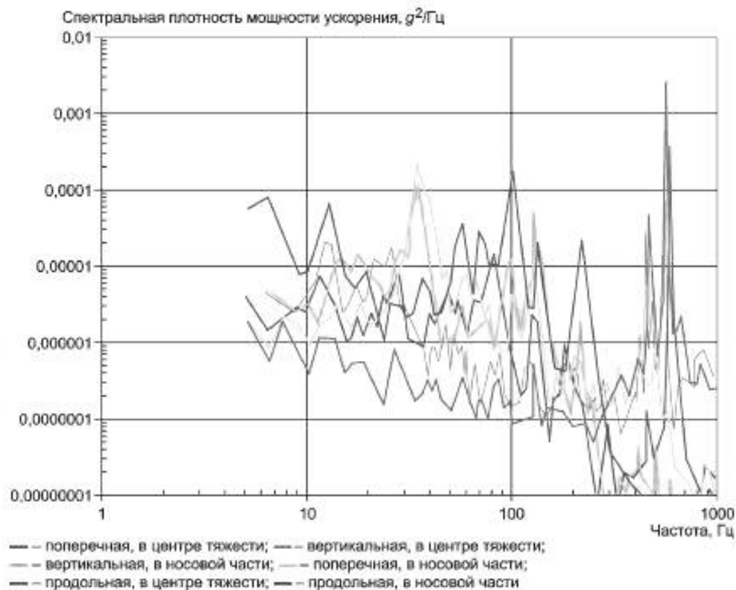
Рисунок 7 — Измерения вибрации на самолете Tristar (режим 10 — см. таблицу 1)
