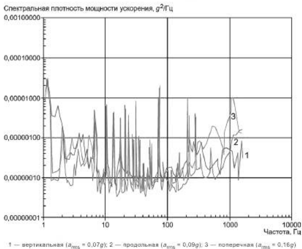
Рисунок 26 — Измерения вибрации на самолете DC8 (крейсерский режим)
