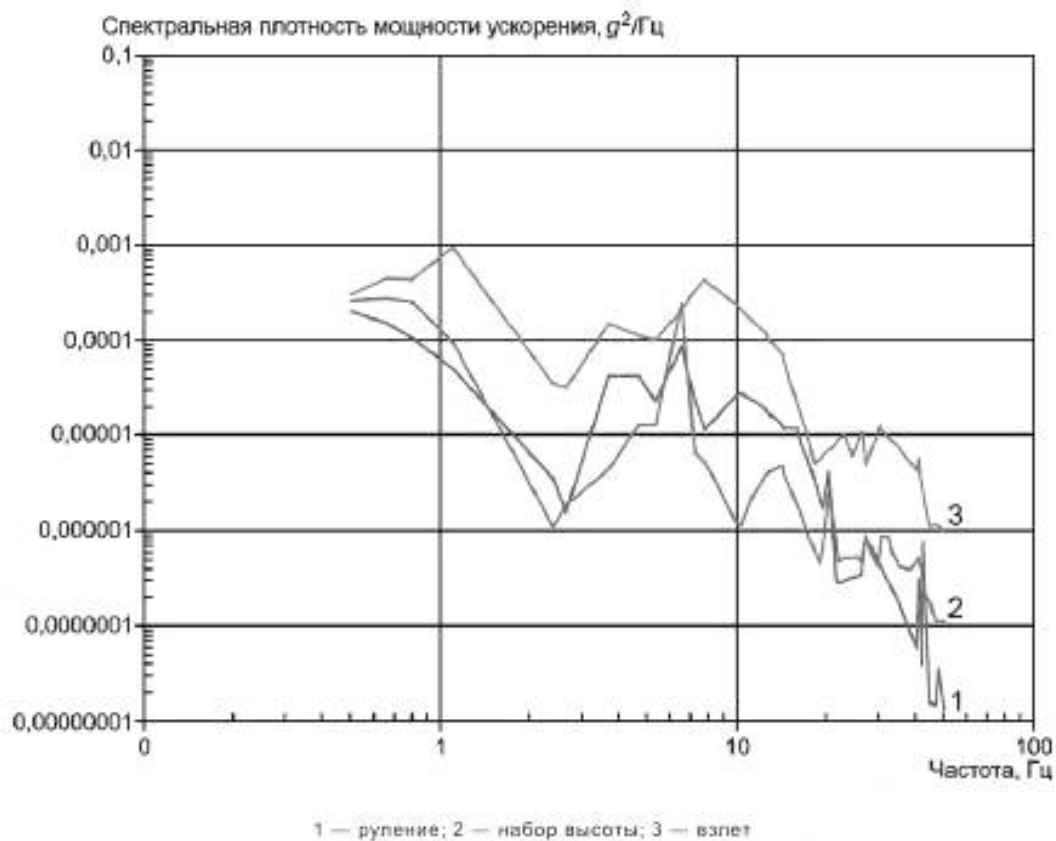
Рисунок 22 — Измерение V1 (см. таблицу 6) на поддоне самолета Boeing 747
