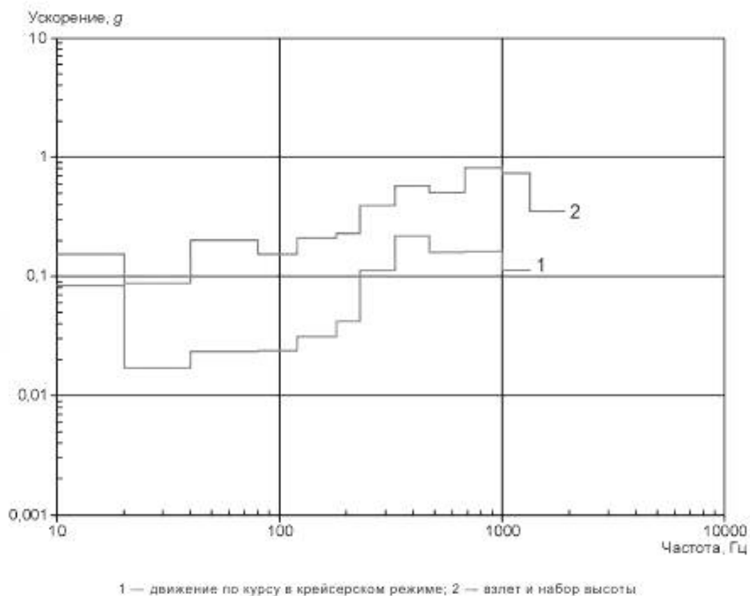
Рисунок 27 — Условия динамических воздействий (пиковые значения ускорения в полосах частот) для самолетов NC-135, C-141, C-5A согласно [9]
