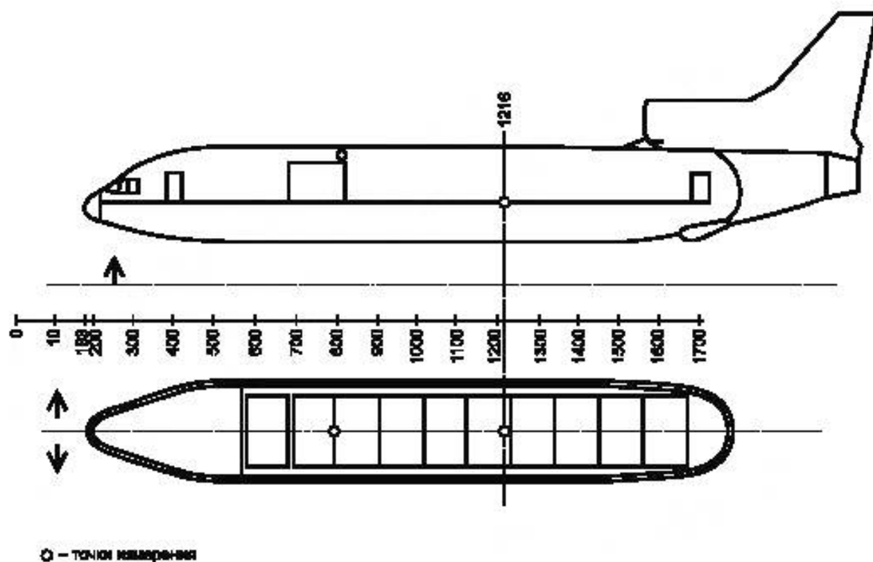
Рисунок 1 — Схематическое изображение самолета Tristar
