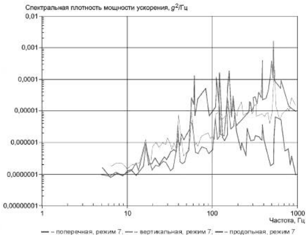
Рисунок 10 — Измерения вибрации на самолете Tristar (датчик в центре тяжести, крейсерский режим)
