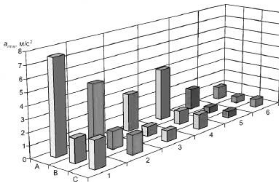
А — испытательный полигон; В — шоссе; С — обычная дорога; 1 — грузовой автомобиль, ось Z; 2 — прицеп, ось Z; 3 — полуприцеп, ось Z; 4 — грузовой автомобиль, оси X, Y; 5 — прицеп, оси X, Y; 6 — полуприцеп, оси X, Y; a_{rms} — среднеквадратичное значение ускорения
