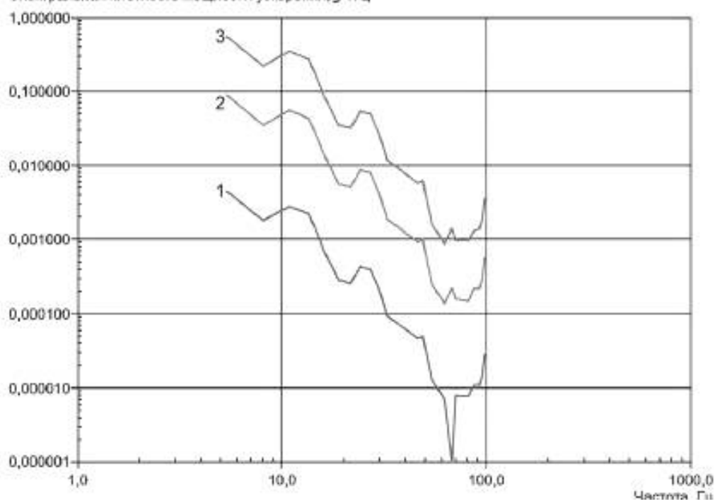
Спектральная плотность мощности ускорения, g^2/Гц
