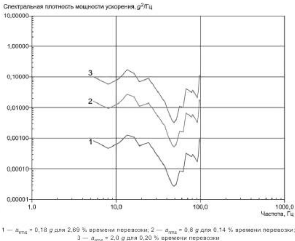
Рисунок 54 — Тестовые воздействия в поперечном направлении по SRETS [три уровня жесткости испытаний по перемещению: высокий ( d_{p-p} = 19,7 мм), средний ( d_{p-p} = 7,9 мм) и низкий ( d_{p-p} = 1,8 мм)] на основе спектра и среднеквадратичного значения a_{rms}
