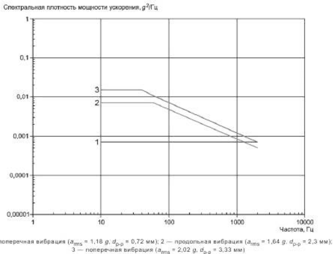
Рисунок 55 — Тестовые воздействия по [17]
