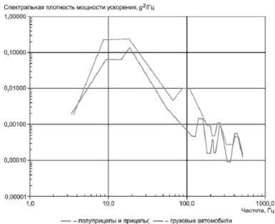
Рисунок 29 — Огибающая спектров по измерениям Холпе и Герока
