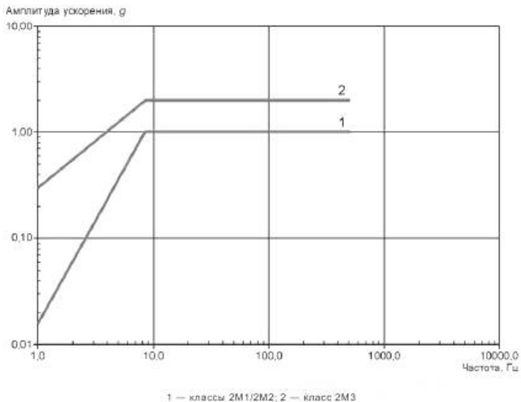
Рисунок 64 — Тестовые воздействия [25] (гармоническая вибрация)
