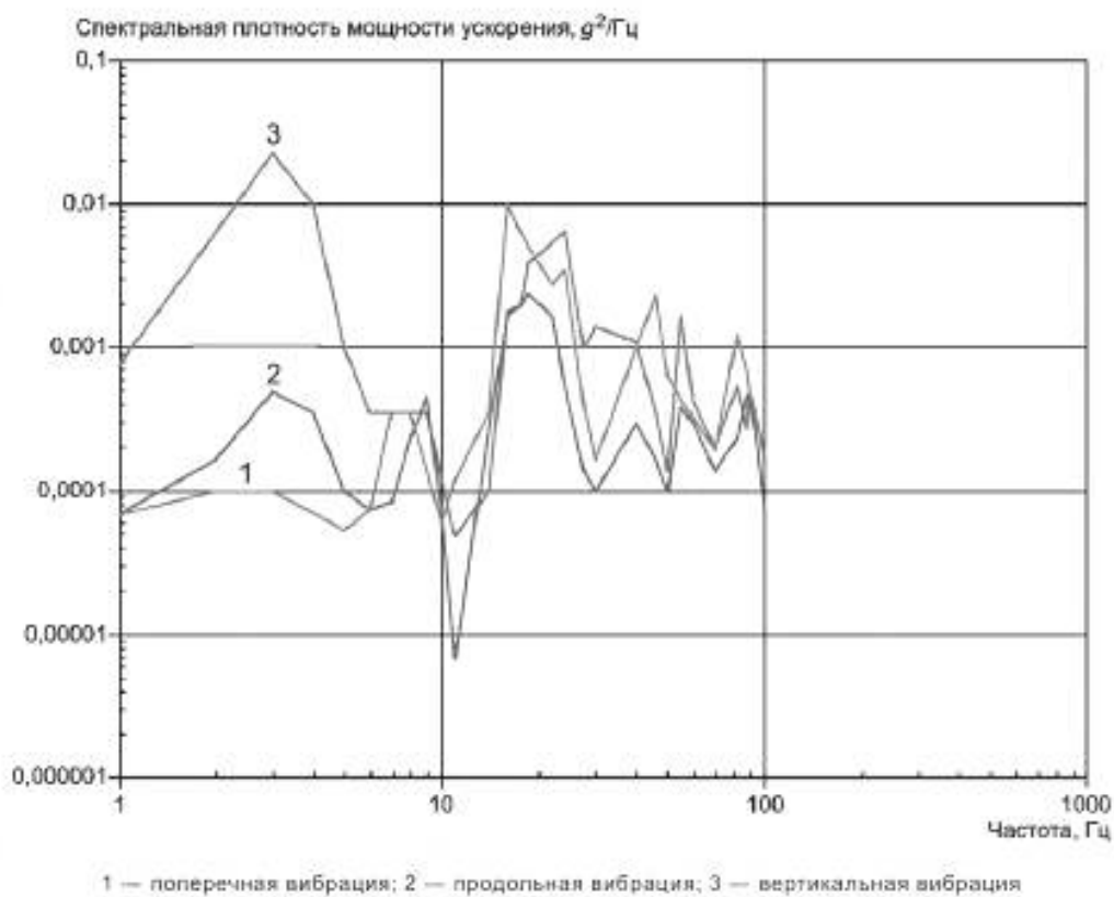
Рисунок 46 — Данные измерений вибрации на прицепе с листовыми рессорами, перевозящим груз массой 18 144 кг со скоростью 88 км/ч по бетонному шоссе по [13]
