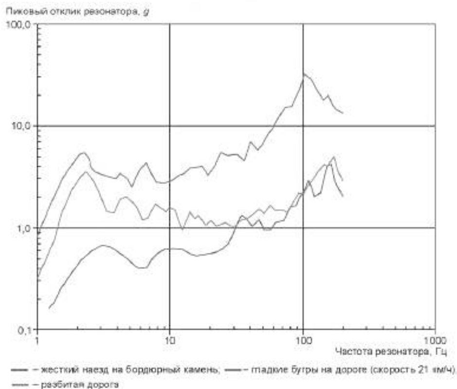
Рисунок 27 — Ударные спектры по измерениям CEEES (добротность Q = 10 )
