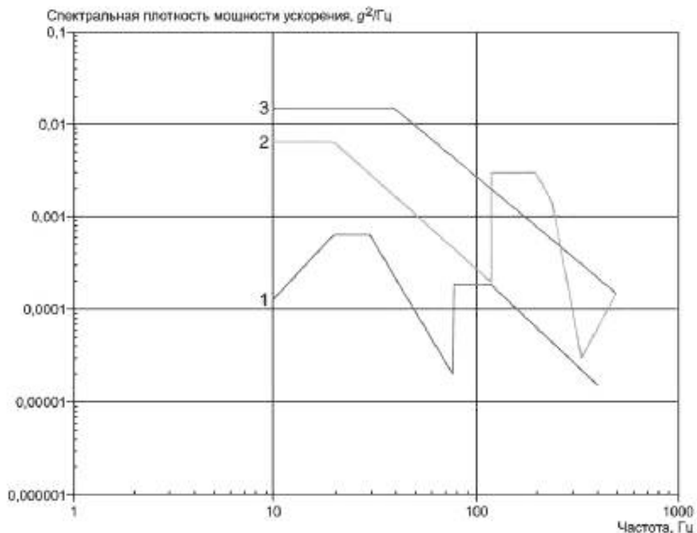
Рисунок 43 — Тестовые воздействия (длительность 60 мин. на 1600 км) по [10]
