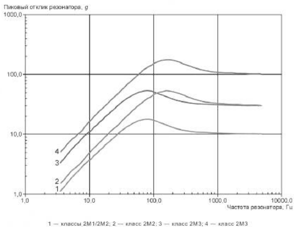
Рисунок 65 — Тестовые воздействия МЭК 60721-3-2:1997 (ударные спектры)
