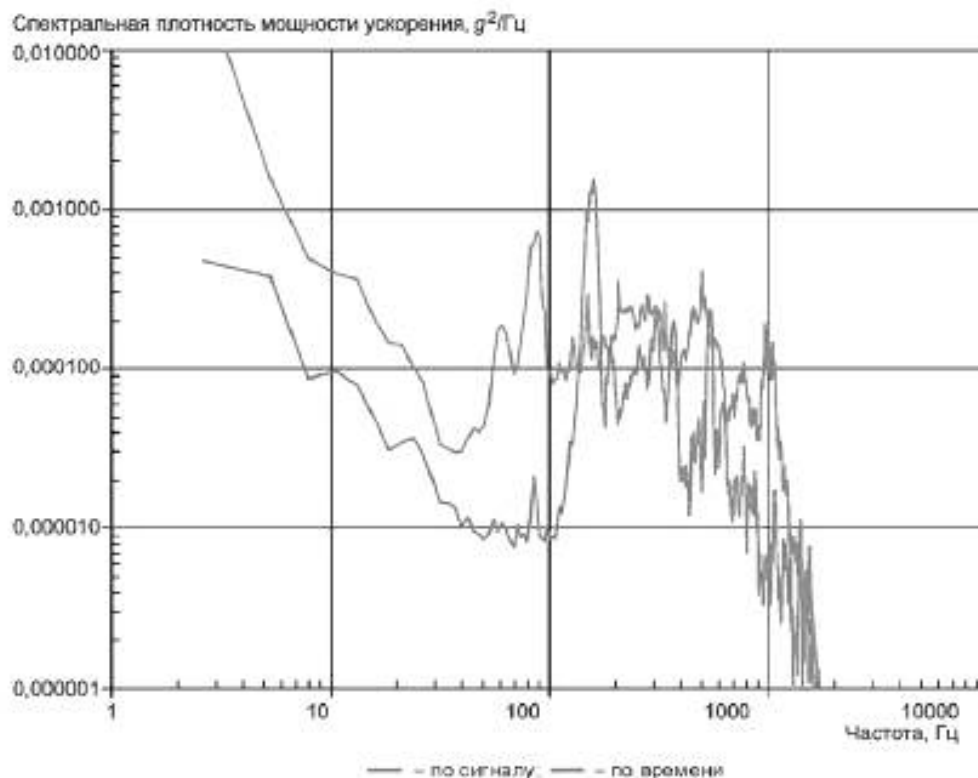
Рисунок 12 — Сравнение результатов измерений программы SRETS (усредненные спектры ускорения в вертикальном направлении) по сигналу ( a_{rms} = 0,47 \text{ g} ) и по времени ( a_{rms} = 0,28 \text{ g} ) без оповещения водителей о цели испытаний
