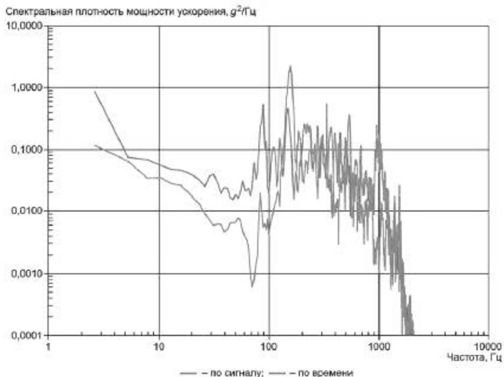
Рисунок 13 — Сравнение результатов измерений программы SRETS (оглабляющие спектры ускорения в вертикальном направлении) по сигналу ( a_{rms} = 9,0 \text{ g} ) и по времени ( a_{rms} = 8,9 \text{ g} ) без оповещения водителей о цели испытаний
