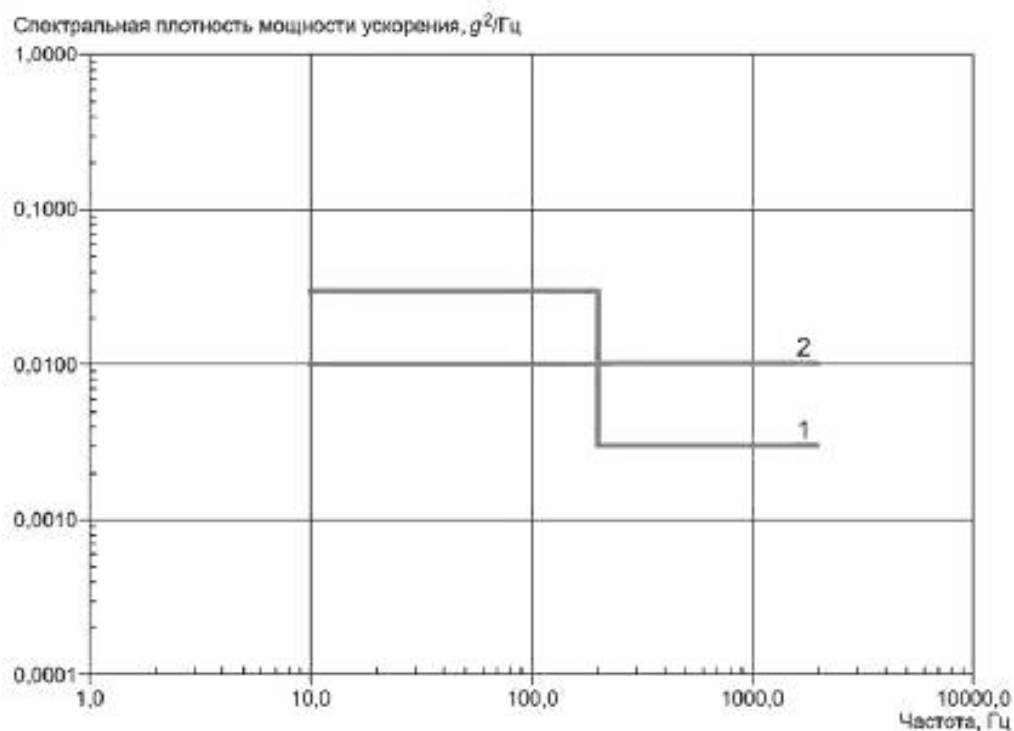
Рисунок 60 — Тестовые воздействия по [20]
