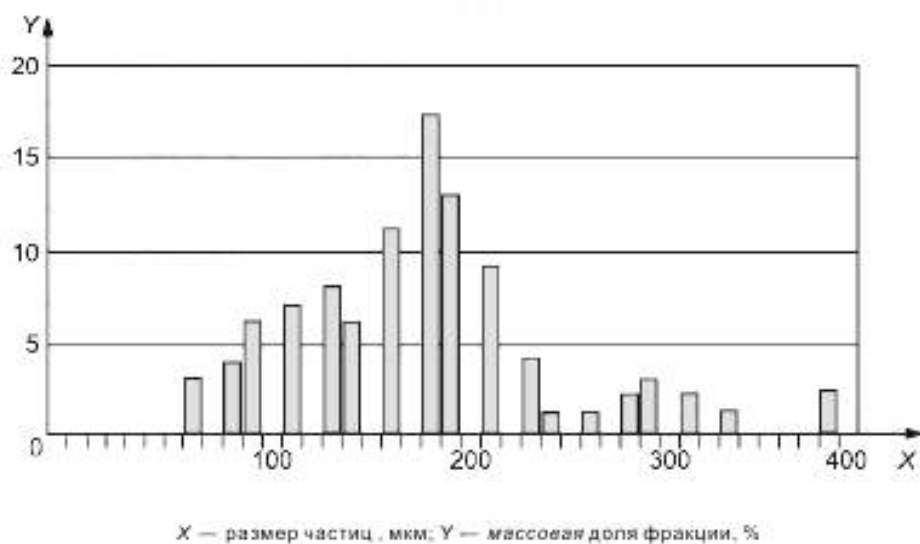
Рисунок А.2 — Распределение частиц порошка ПКЛ, полученного с помощью измельчителя и затем просеянного
