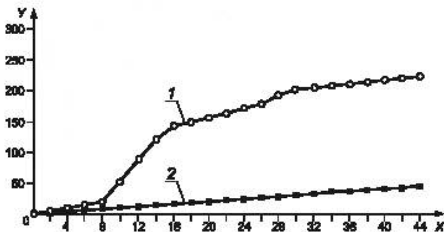
Рисунок В.1 — Кривая выделения диоксида углерода
