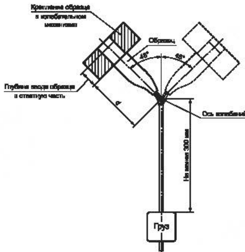
Рисунок 2 — Схема перемещения испытываемого образца неразъемного соединителя во время испытания прочности на изгиб
