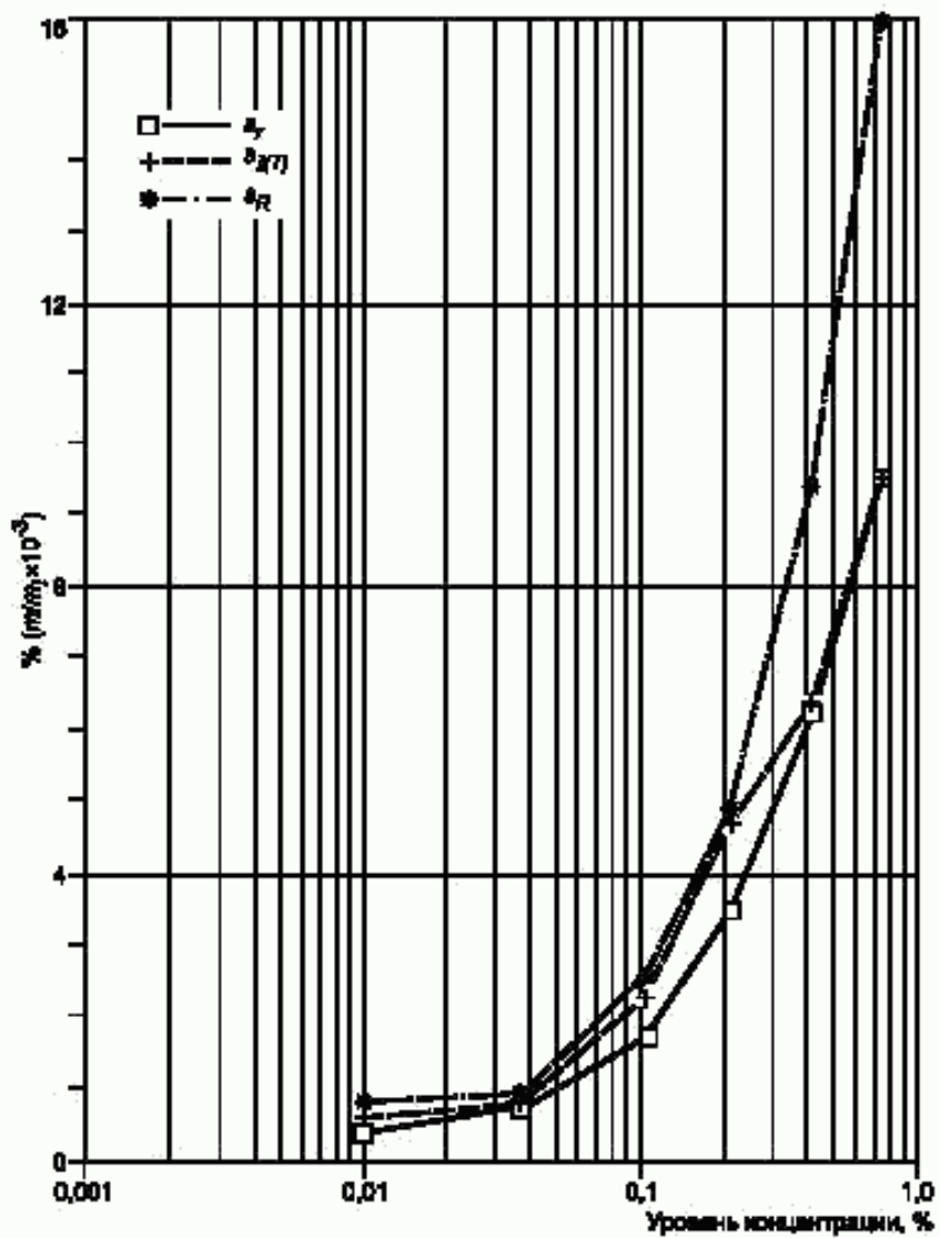
Рисунок D.3 — Содержание ванадия в стали. Стандартные отклонения повторяемости s_r , промежуточной прецизионности с изменяющимся фактором времени s_{R(T)} и воспроизводимости s_R как функции уровня концентрации
