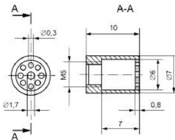
Рисунок Г.8 — Стабилизатор пламени горелки
