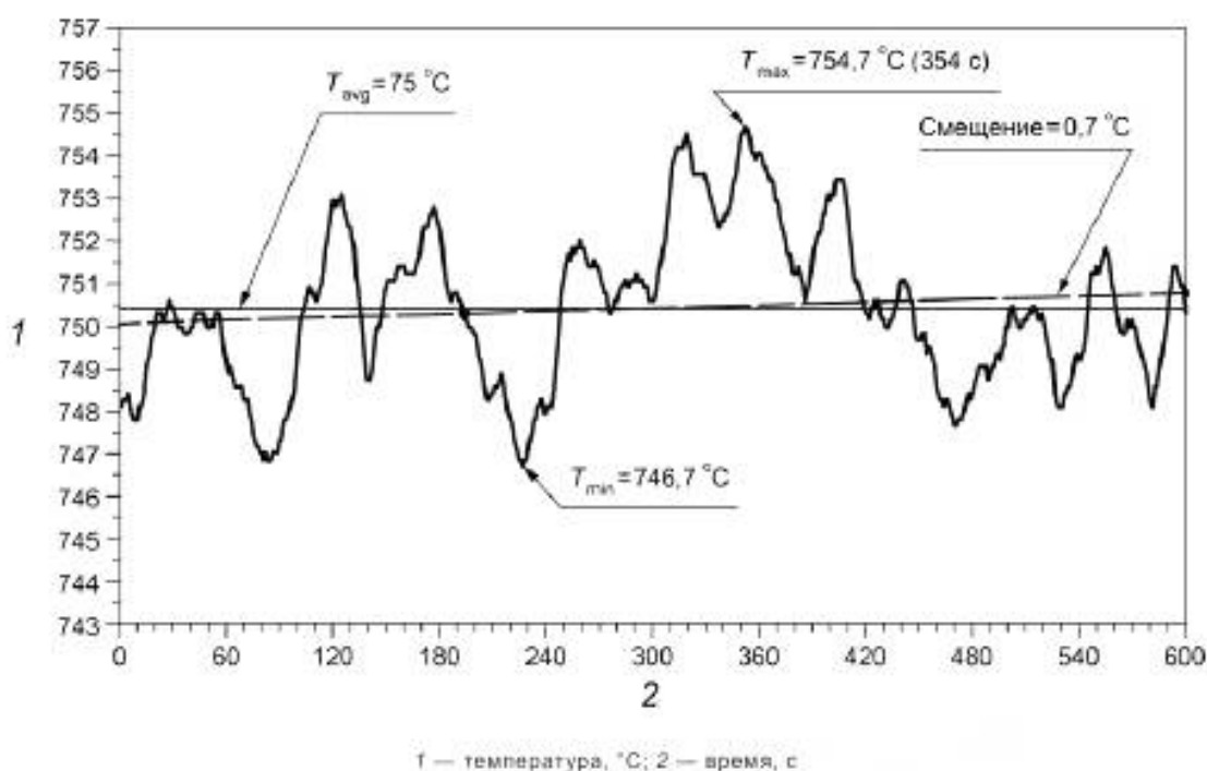
Рисунок Б.1 — Пример стабилизации начальной температуры
