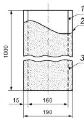
Рисунок В.3 — Схема определения длины повреждения образца
