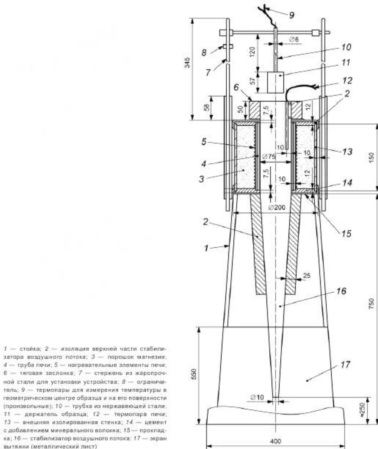
Рисунок А.1 — Типовое расположение оборудования установки для испытаний по методу I
