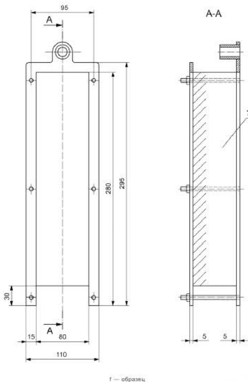
1 — образец Рисунок Г.2 — Держатель образца для испытаний однослойных материалов
