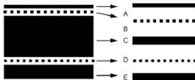
Рисунок Ж.1 — Многослойный материал
