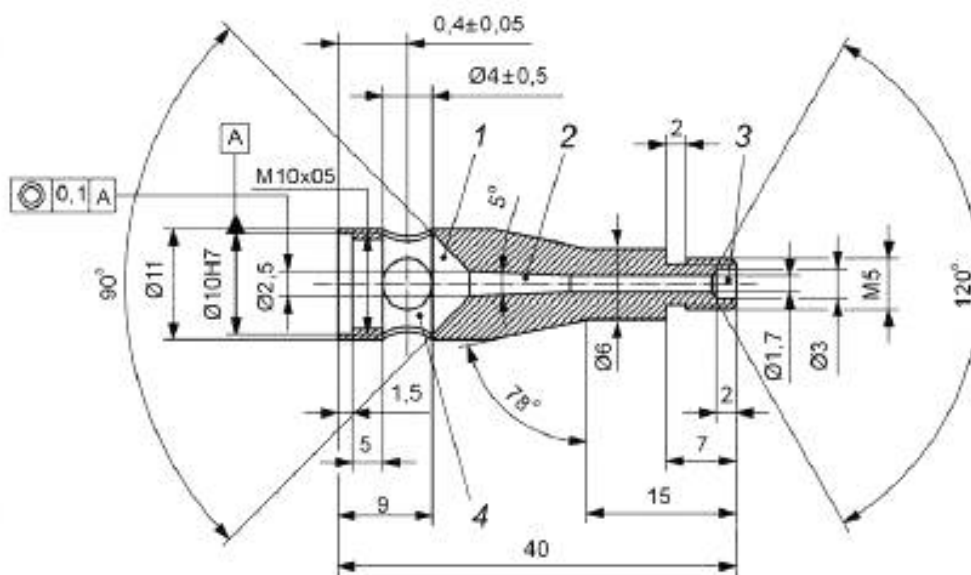
Рисунок Г.8 — Стабилизатор пламени горелки
