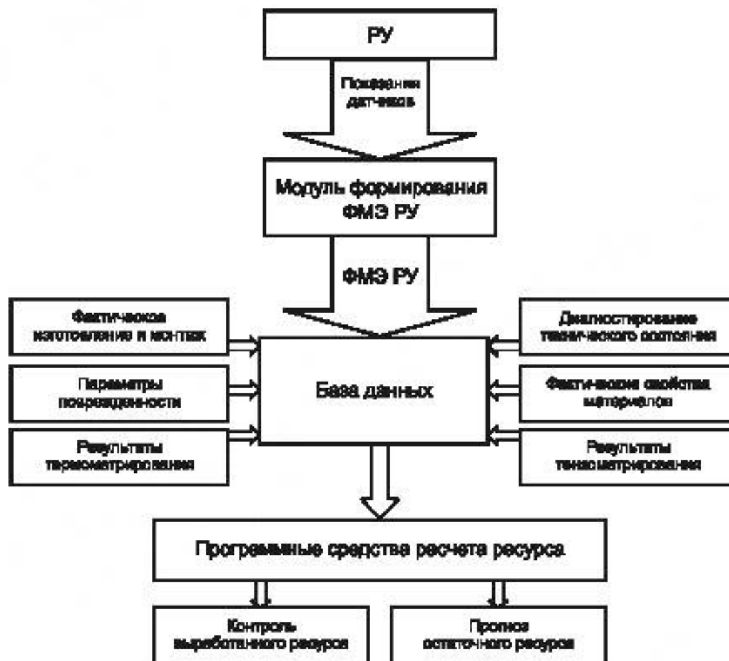
Рисунок 1 — Принципиальная схема организации ЭМР
