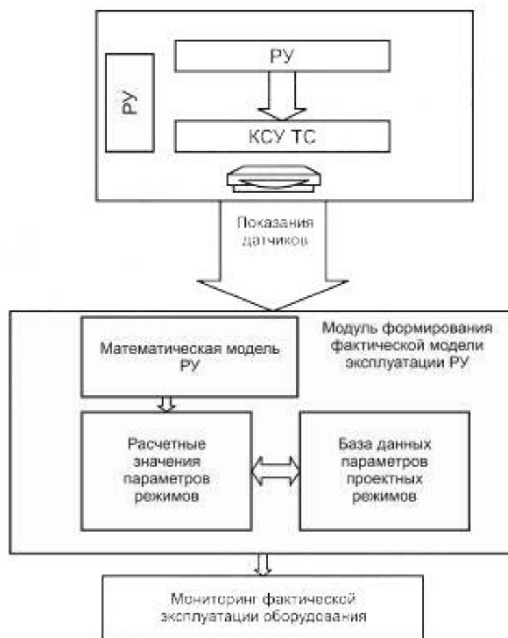
Рисунок 4 — Принципиальная схема работы модуля формирования ФМЭ РУ
