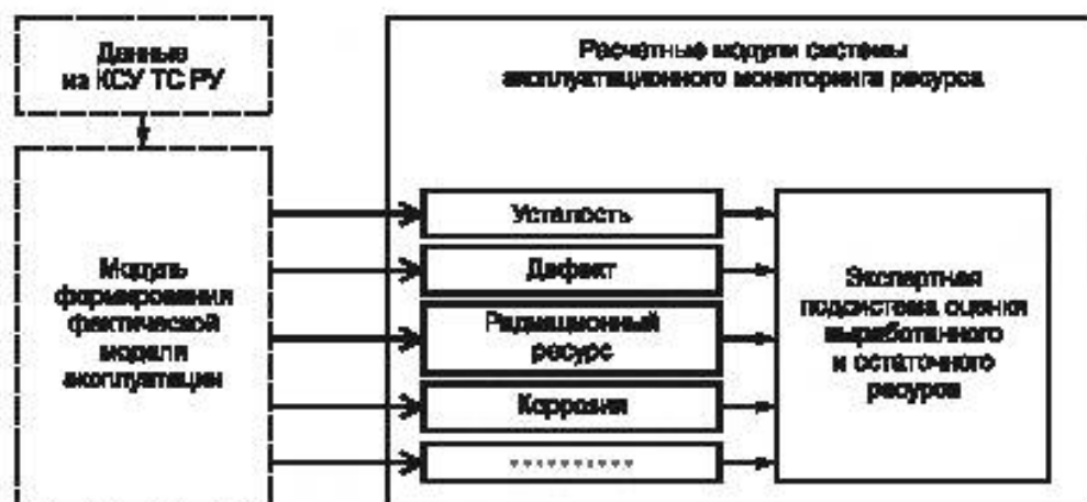
Рисунок 6 — Общая схема взаимодействия расчетных модулей системы СЭМР
