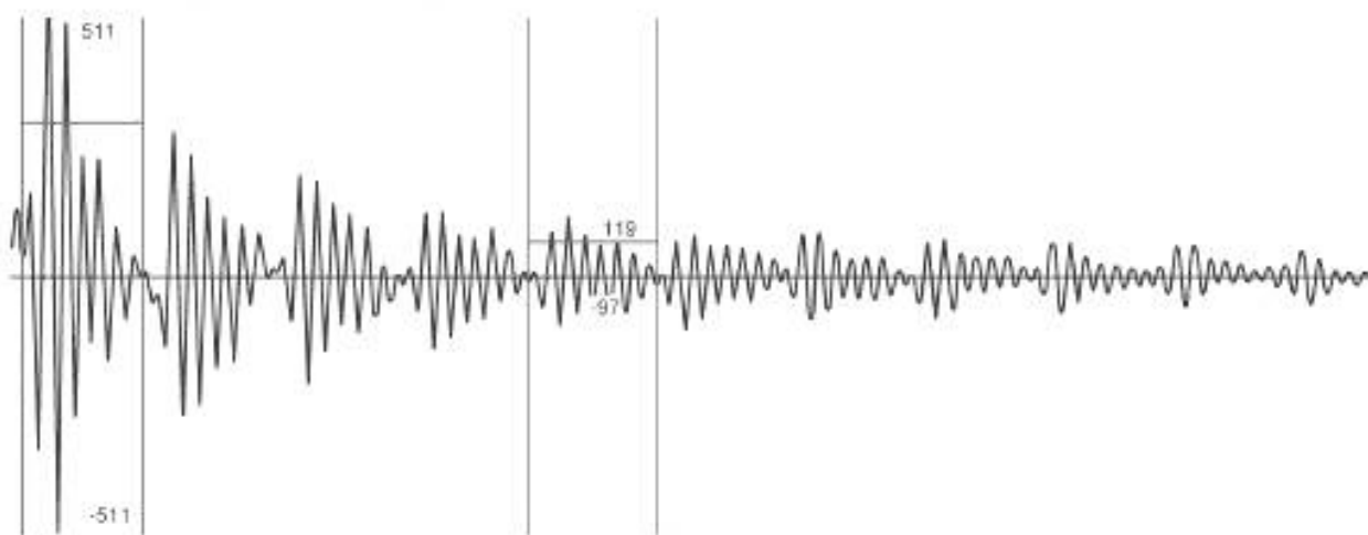
Рисунок 5 — Осциллограмма продольных импульсов с приемлемым соотношением «сигнал/шум»
