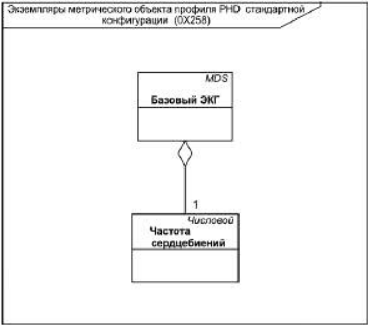
Рисунок 5 — Профиль ЧСС. Стандартная конфигурация (0x258). Метрические объекты
