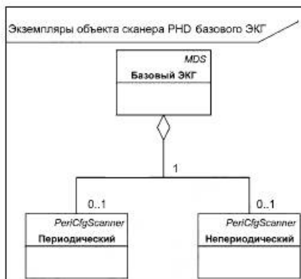
Рисунок 8 — Базовый ЭКГ (от 1 до 3 отведений). Модель сканера
