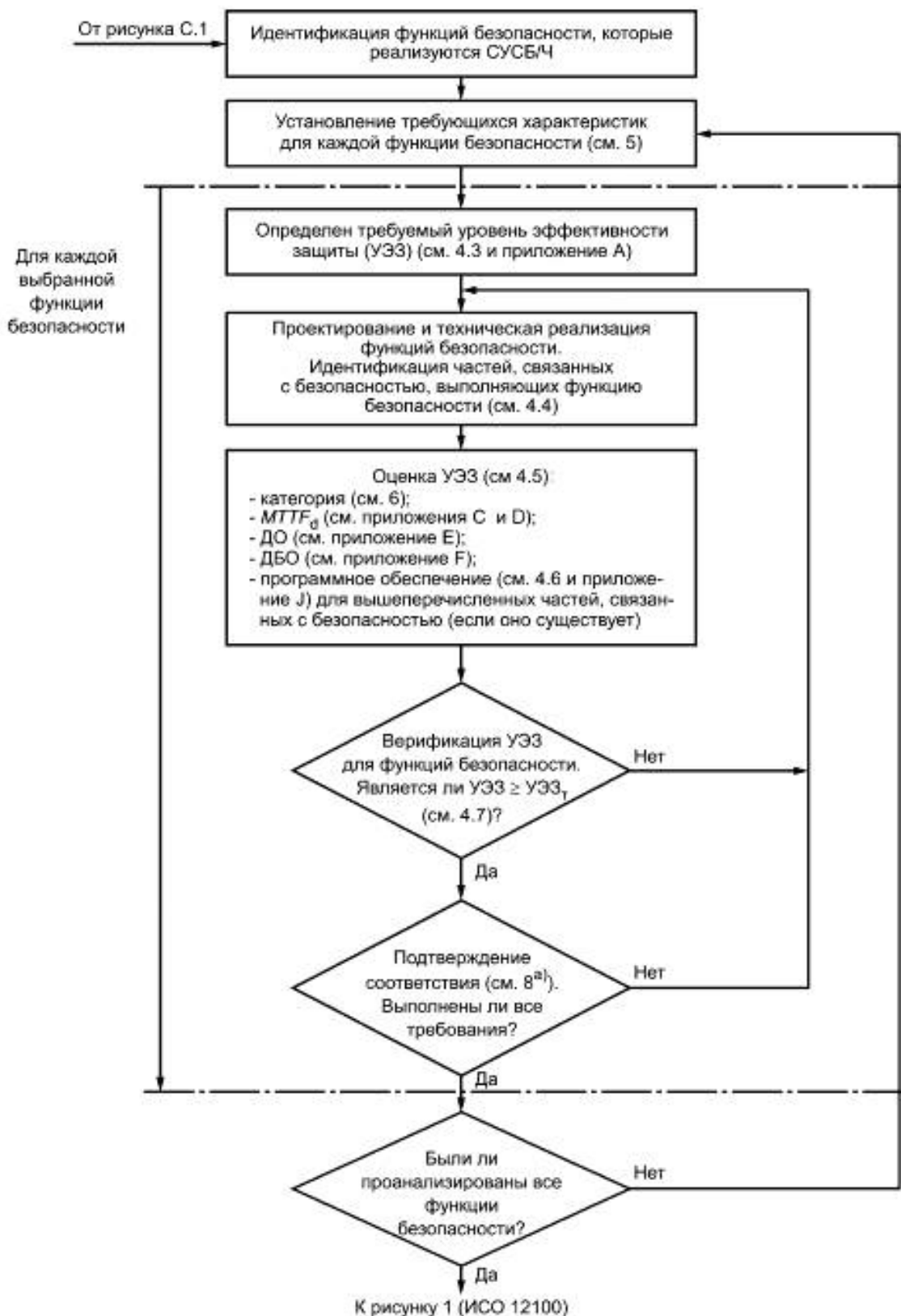
Рисунок С.2 — Блок-схема обобщенного процесса. Итеративный процесс проектирования связанных с безопасностью частей систем управления (СУСБ/Ч) (ИСО 13849-1:2006, рисунок 3)
