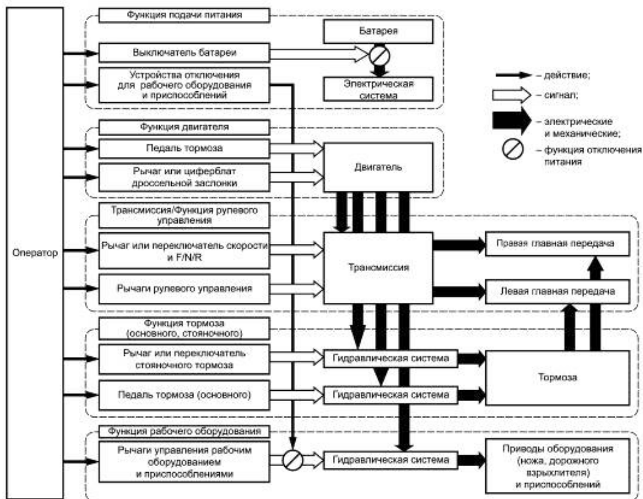
Рисунок А.2 — Бульдозер на гусеничном ходу
