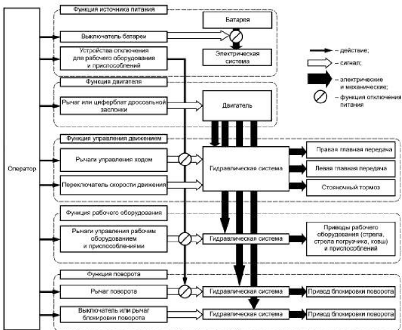
Рисунок А.3 — Экскаватор на гусеничном ходу
