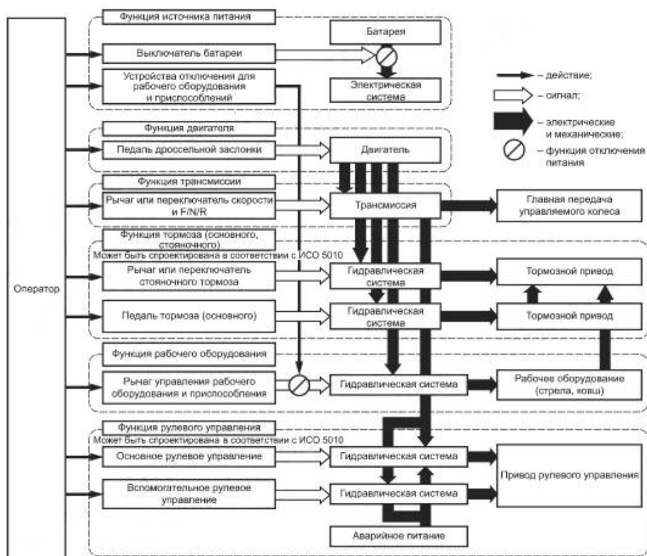
Рисунок А.5 — Шарнирно-сочлененный колесный погрузчик
