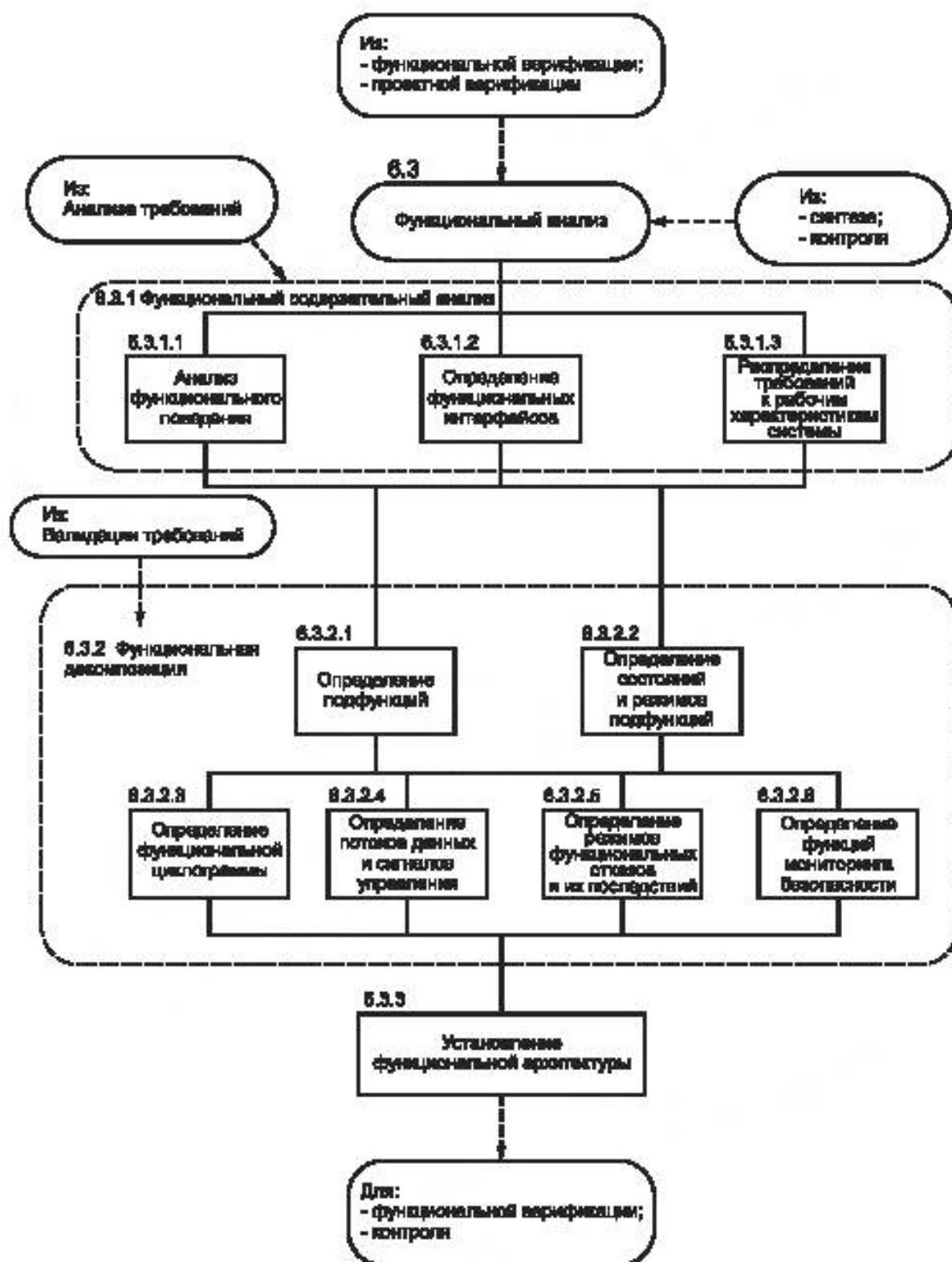
Рисунок 12 — Блок-схема процесса функционального анализа
