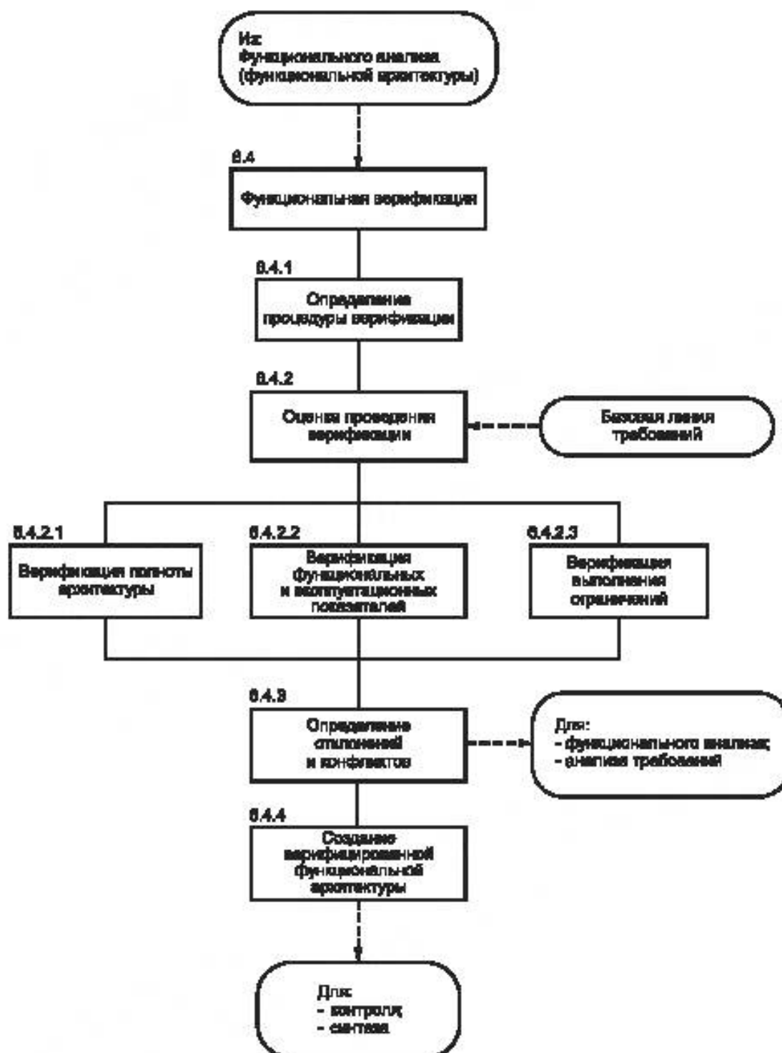
Рисунок 13 — Функциональная верификация
