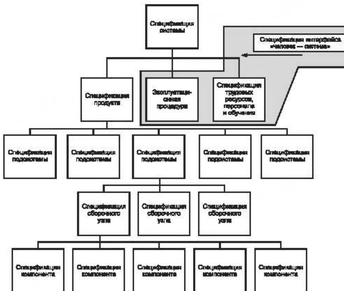
Рисунок 5 — Блок-схема древа спецификаций
