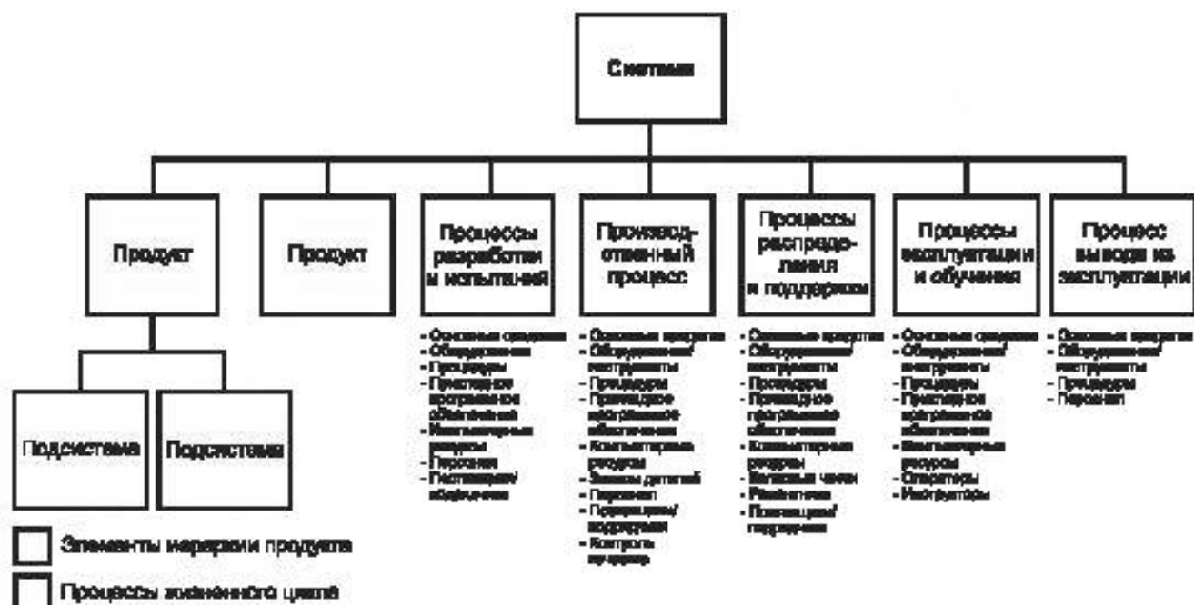
Рисунок 3 — Определение процессов жизненного цикла
