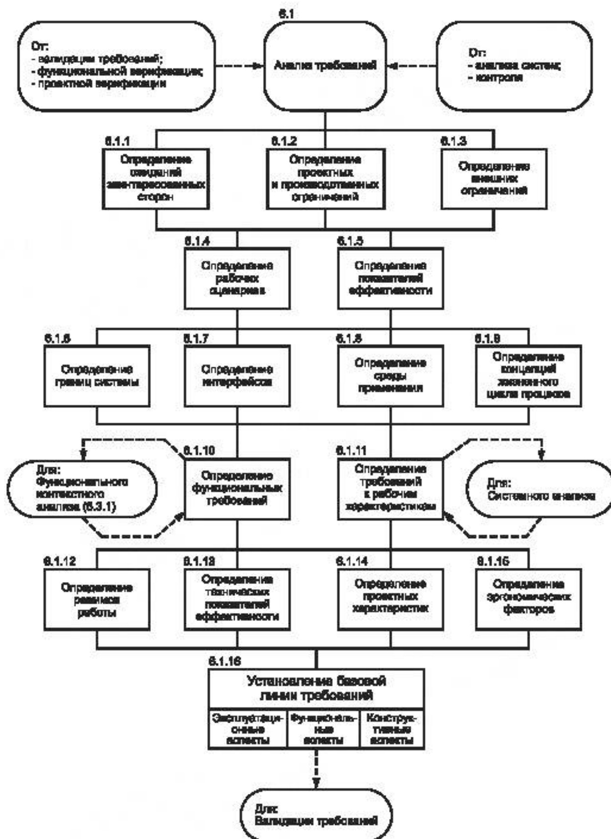
Рисунок 10 — Анализ требований
