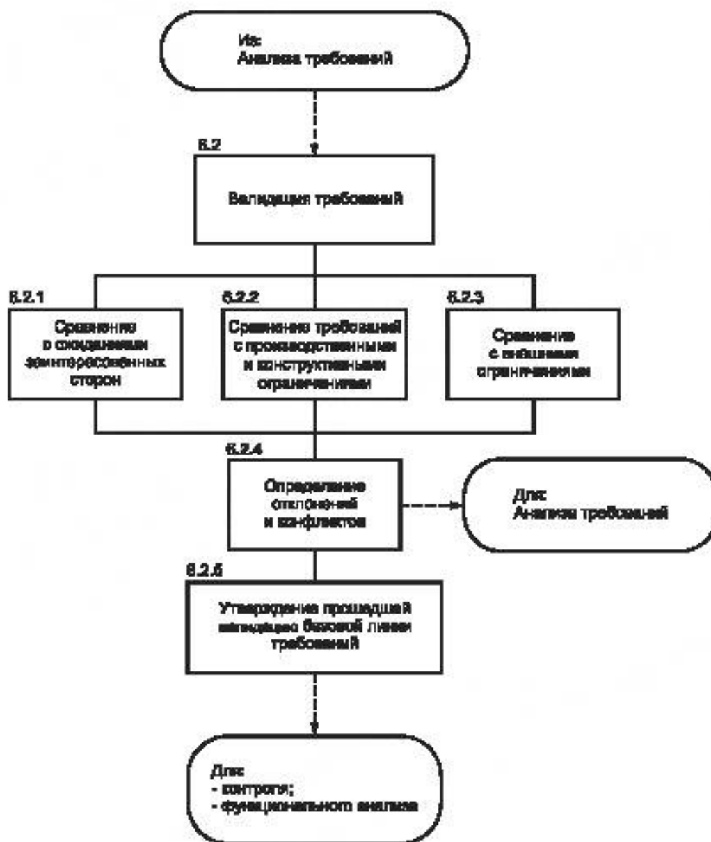
Рисунок 11 — Валидация требований
