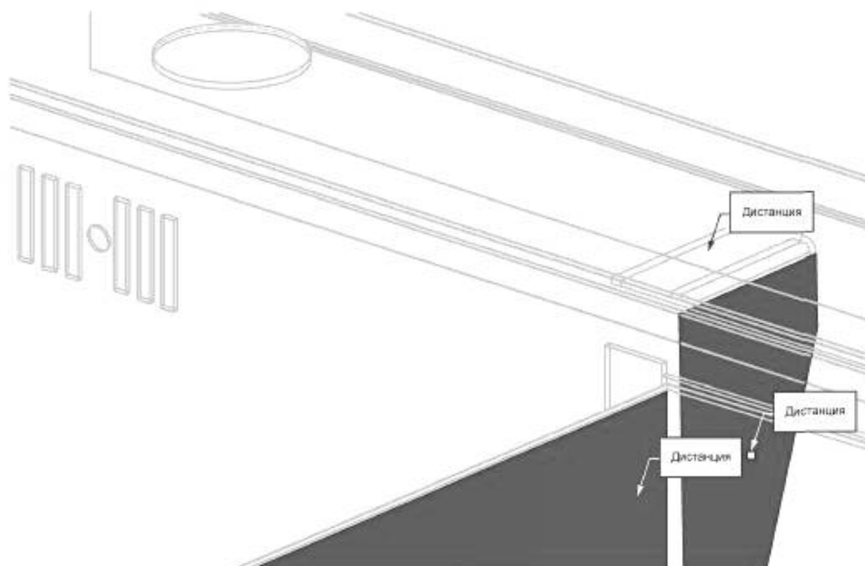
Рисунок 14 — CAD-база знаний — позиционирование монтажного кронштейна [ограничение (выделено цветом): позиция «лицом к лицу»]
