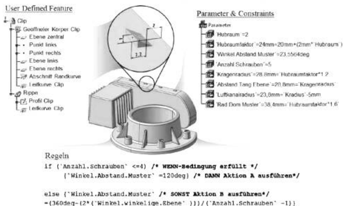
Рисунок 19 — CAD-модель дроссельной заслонки (с сохраненными знаниями)
