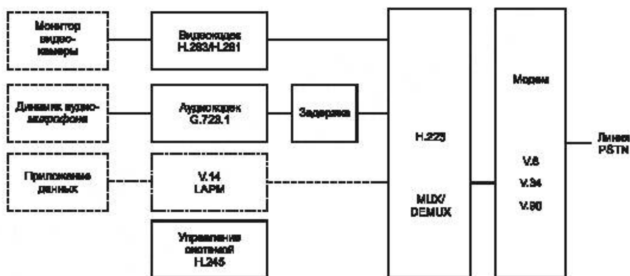
Рисунок 5 — Терминал H.324
