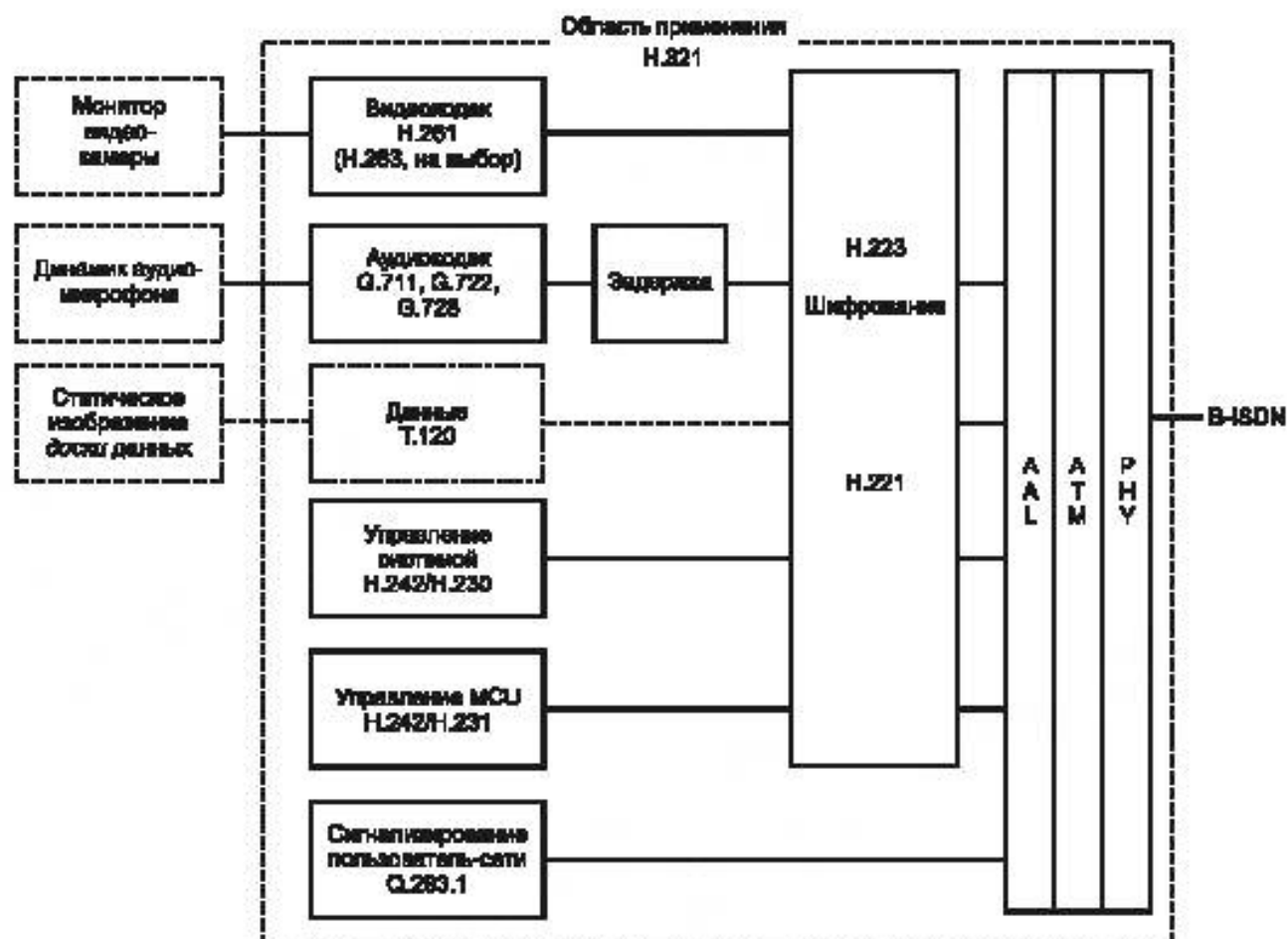
Рисунок 3 — Терминал H.321
