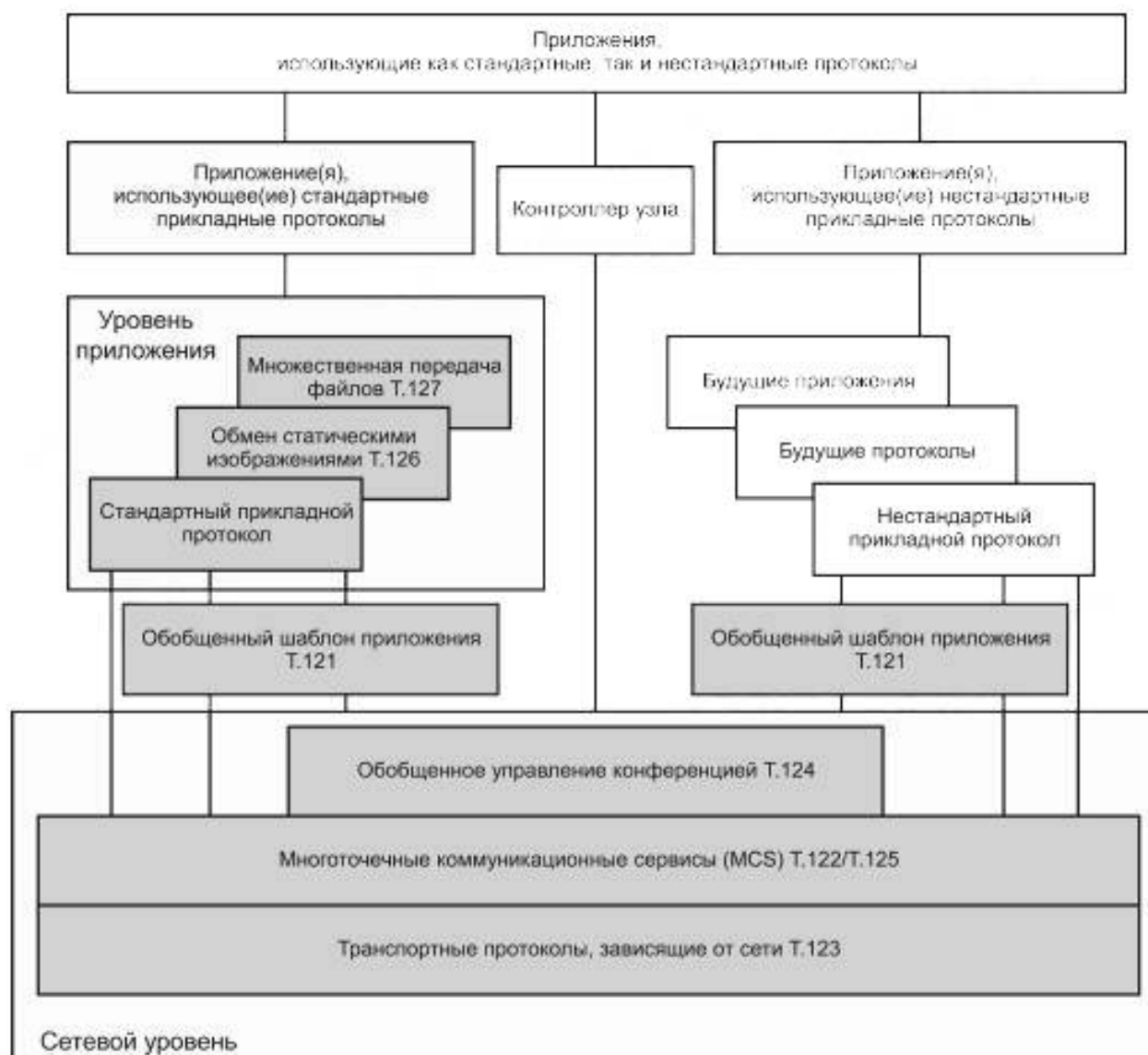
Рисунок 6 — Рекомендации T.120
