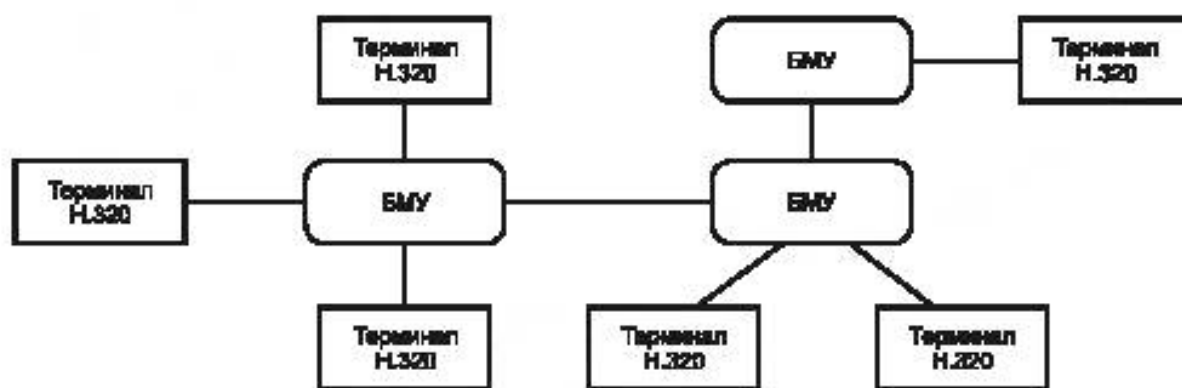
Рисунок 2 — Многоточечная конфигурация
