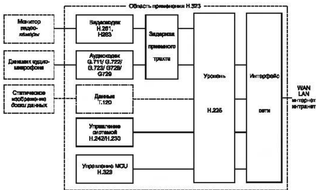
Рисунок 4 — Терминал H.323
