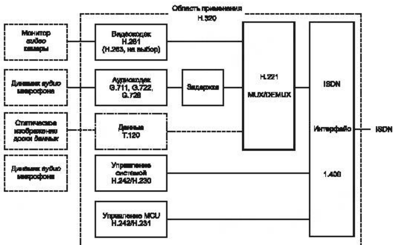
Рисунок 1 — Терминал H.320
