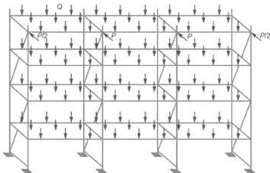
Рисунок 8 — Испытание на воздействие вертикальной нагрузки
