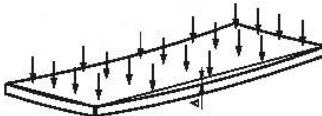
Рисунок 5 — Прогиб полки (балок с полками)
