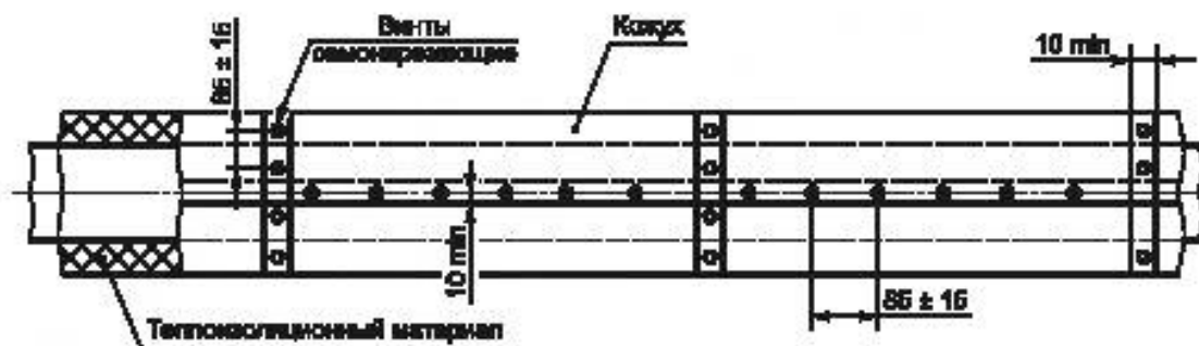
Рисунок 6.5 — Конструкция трубы в теплоизоляции
