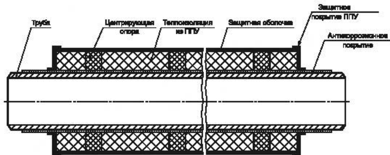
Рисунок 6.1 — Конструкция трубы в теплоизоляции
