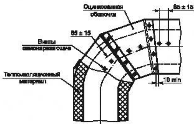
Рисунок 6.6 — Конструкция СДТ в теплоизоляции
