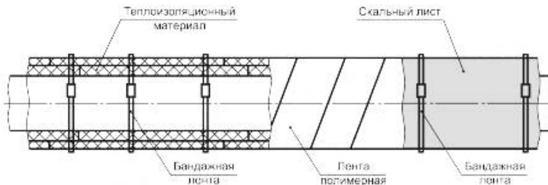
Рисунок 6.7 — Конструкция трубы в теплоизоляции с использованием скорлуп
