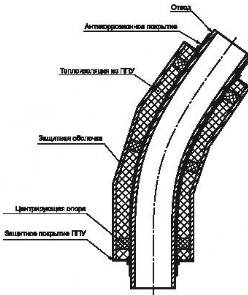
Рисунок 6.2 — Конструкция СДТ в теплоизоляции
