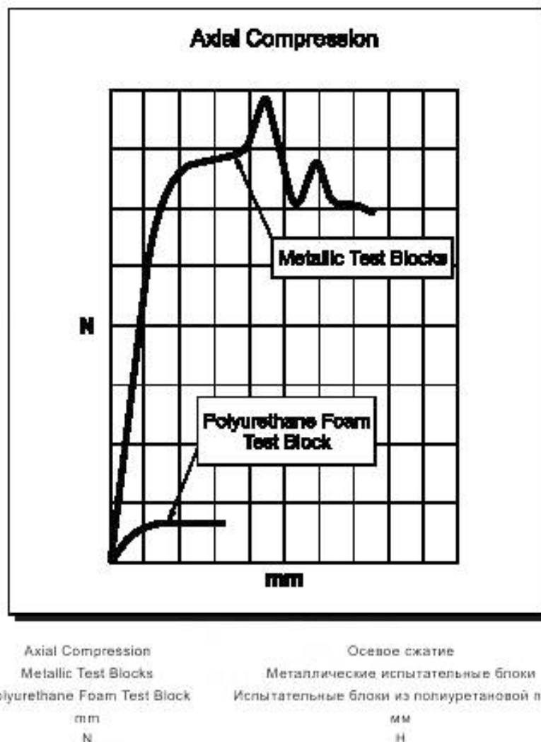
Рисунок 3 — Типичный график «нагрузка—смещение» для сравнения испытуемых образцов в металлических и полиуретановых испытательных блоках
