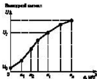
Рисунок 7 — Общий вид градуировочной характеристики
