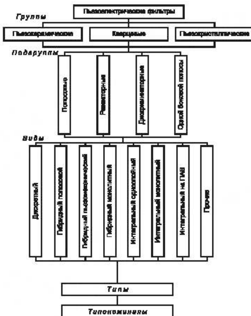
Рисунок 1 — Классификация пьезоэлектрических фильтров
