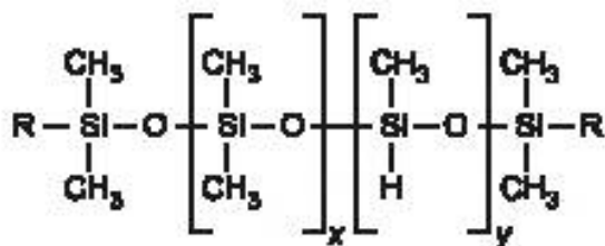
Рисунок 2 — Типичный полимерный сшивающий агент
