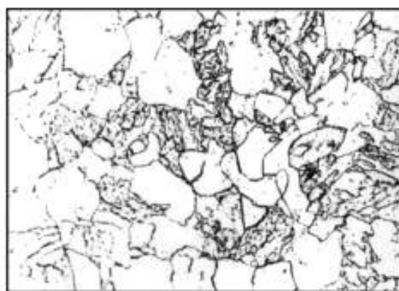
Балл 3, 500 \times , химическое травление
