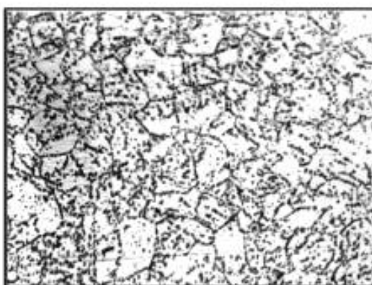
Балл 1, 500 \times , электролитическое травление
