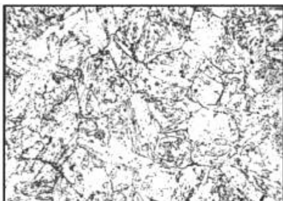
Балл 1, 100 x
