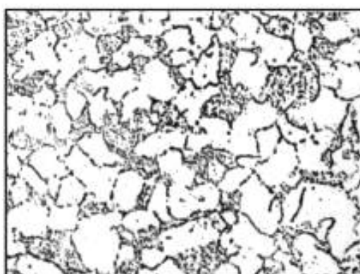
Балл 4, 500 \times , электролитическое травление
