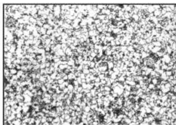
Балл 6, 100 \times , химическое травление
