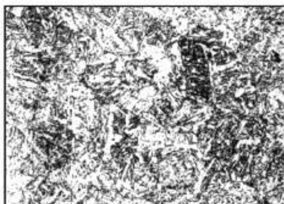
Балл 10, 100 х
