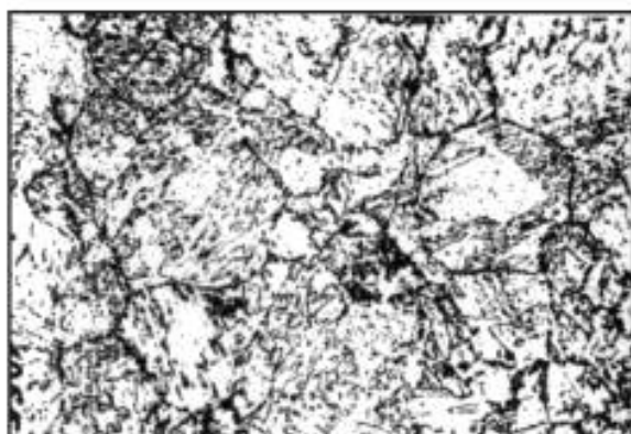
Балл 8, 100 x
