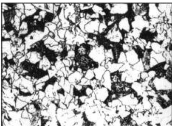
Балл 3, 100 ×
