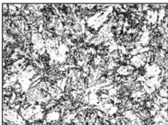
Балл 7, 100 x
