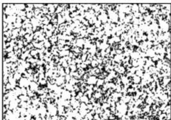
Балл 9, 100 ×
