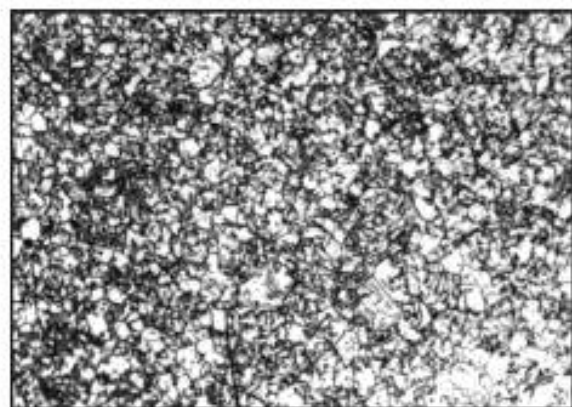
Балл 2, 100 \times , химическое травление
