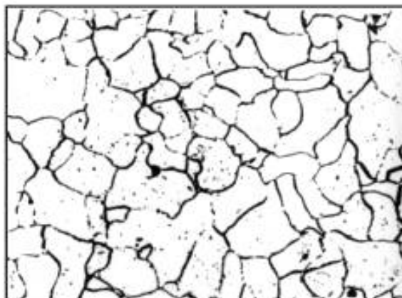
Балл 7, 500 ×
