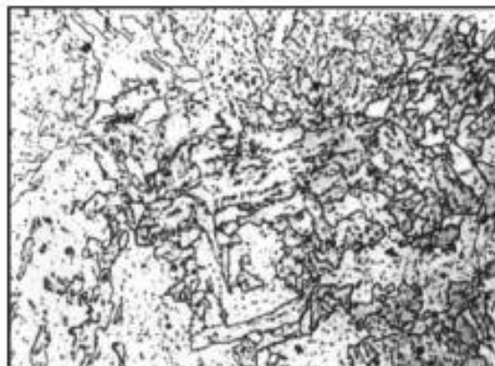
Балл 1, 500 ×
