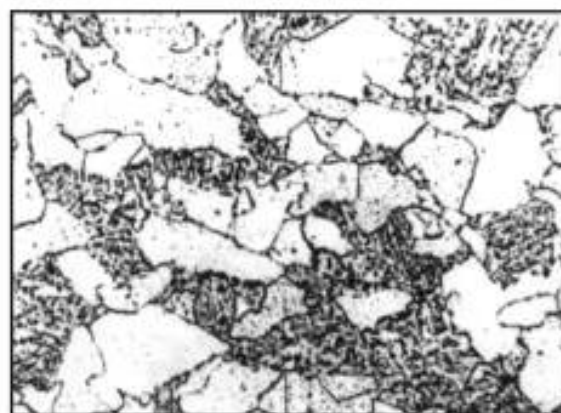
Балл 2, 500 ×
