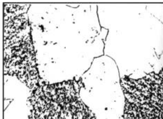
Балл 4, 500 x
