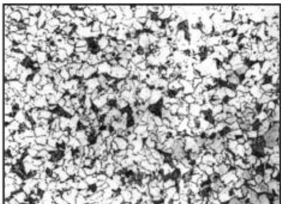
Балл 4, 100 x
