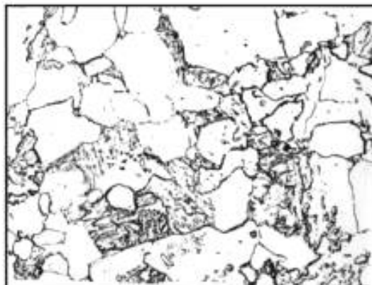
Балл 4, 500 \times , химическое травление
