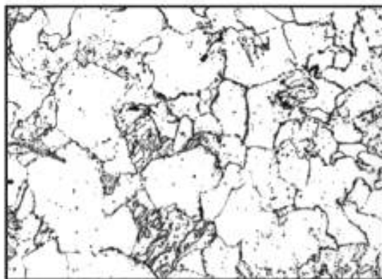
Балл 5, 500 \times , химическое травление
