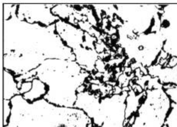
Балл 9, 500 ×
