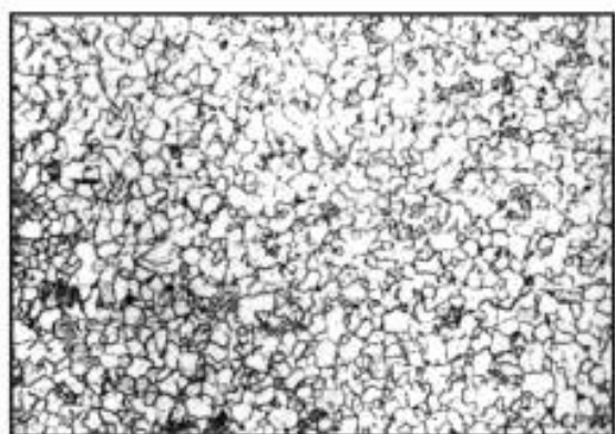
Балл 7, 100 \times , химическое травление
