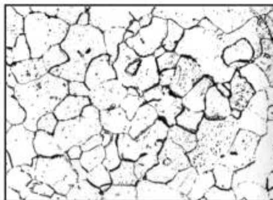
Балл 7, 500 \times , химическое травление
