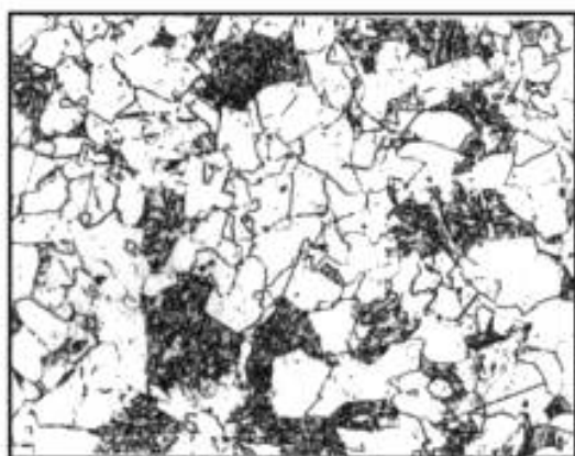
Балл 5, 100 x
