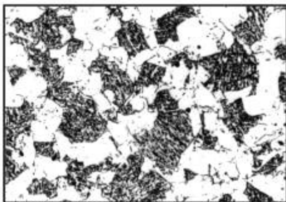
Балл 4, 100 x
