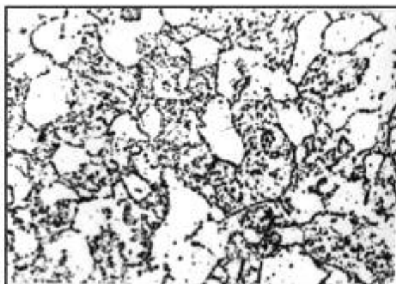
Балл 3, 500 \times , электролитическое травление
