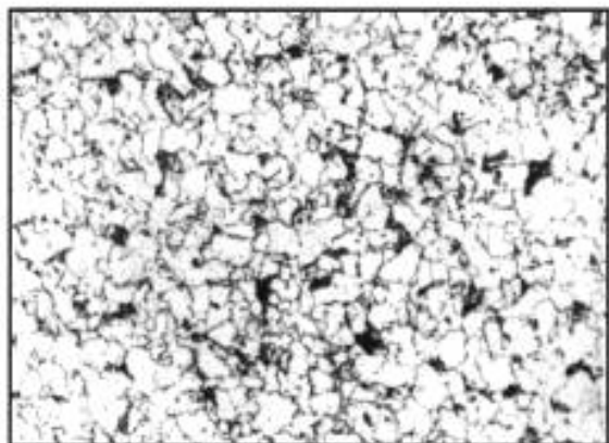
Балл 6, 100 x
