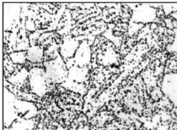
Балл 2, 500 \times , электролитическое травление
