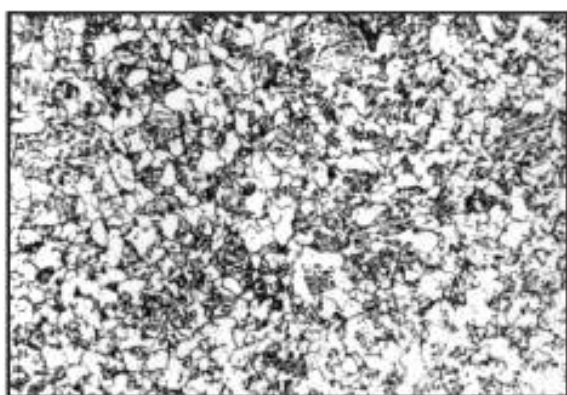
Балл 3, 100 \times , химическое травление
