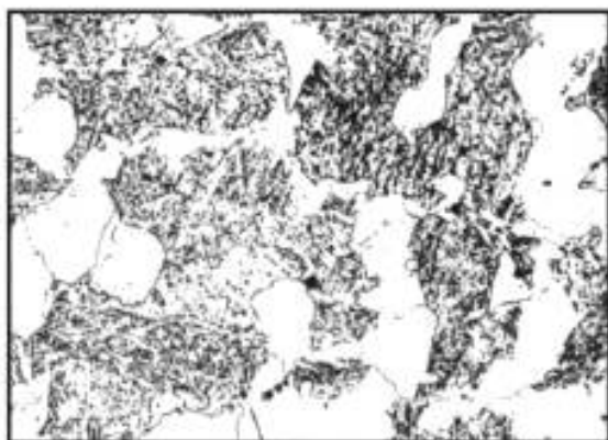
Балл 3, 100 x
