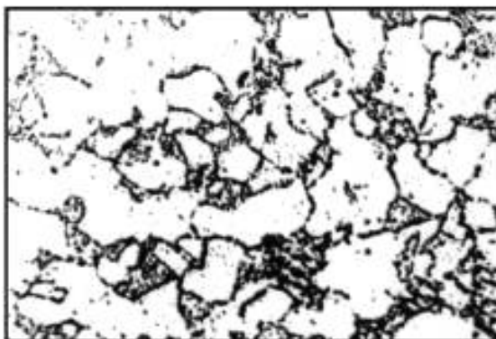
Балл 5, 500 \times , электролитическое травление
