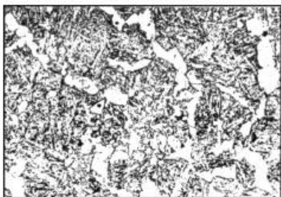
Балл 2, 100 x
