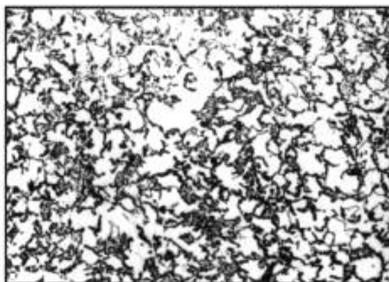
Балл 9, 100 х
