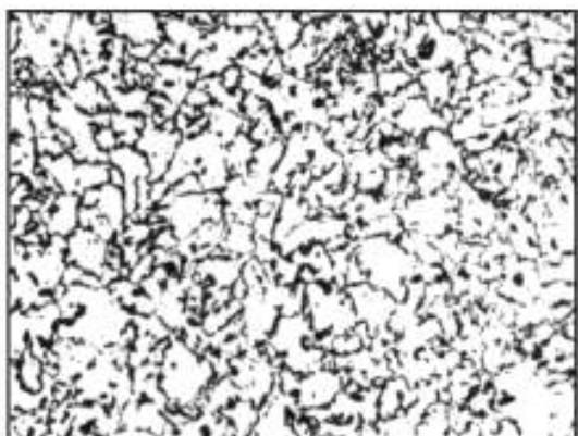
Балл 8, 100 ×
