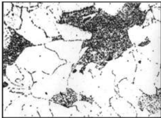
Балл 4, 500 x
