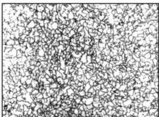
Балл 7, 100 ×
