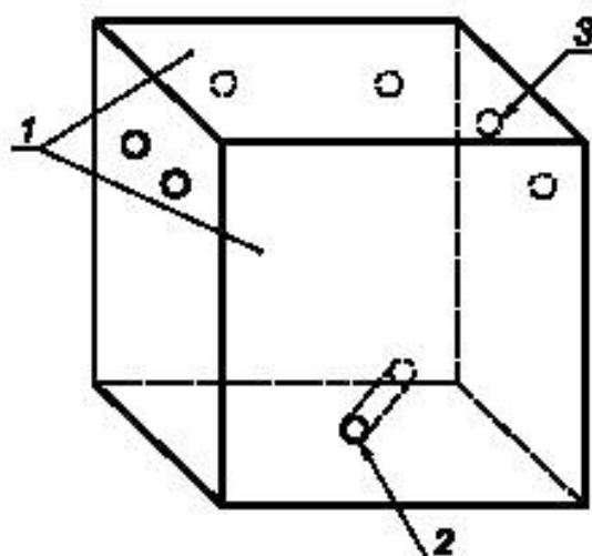
1 — сменные фронтальная и задняя панели; 2 — воздухохранилище; 3 — боковые отверстия (диаметром 10 мм)
