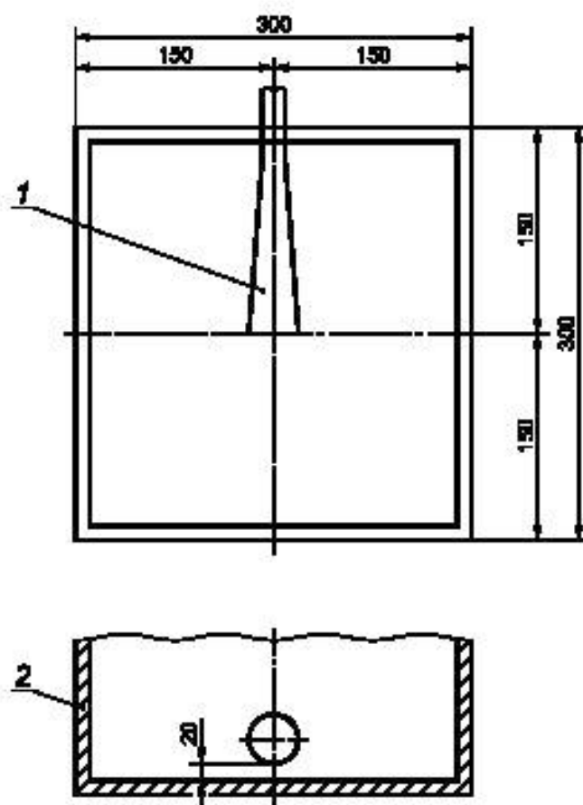
1 — всасывающий зонд воздухохранилища; 2 — изгибающаяся камера
