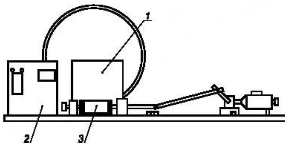
1 — камера для испытаний; 2 — счетчик частиц; 3 — испытательный образец
