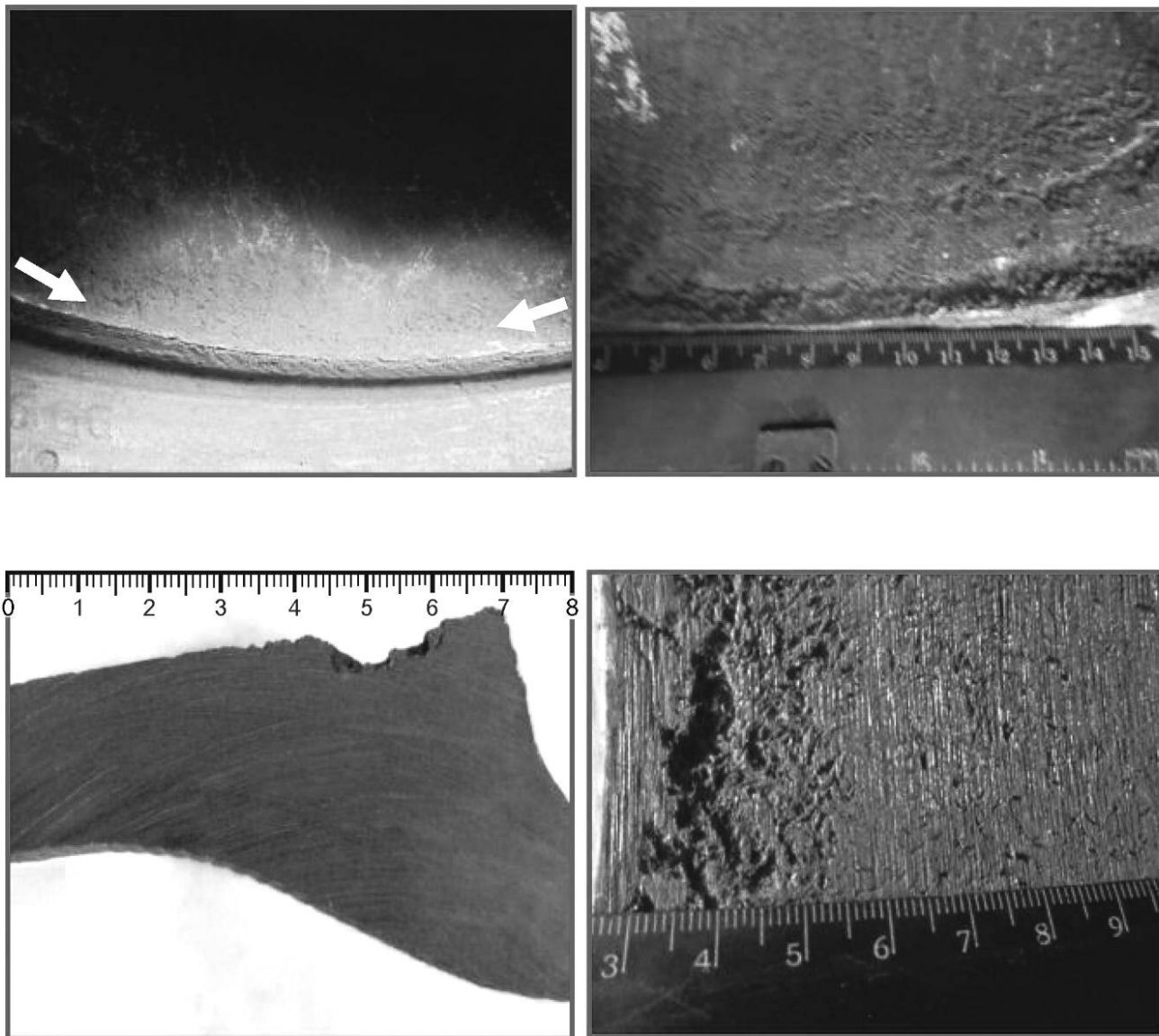
Рисунок Д.4 — Утяжина
