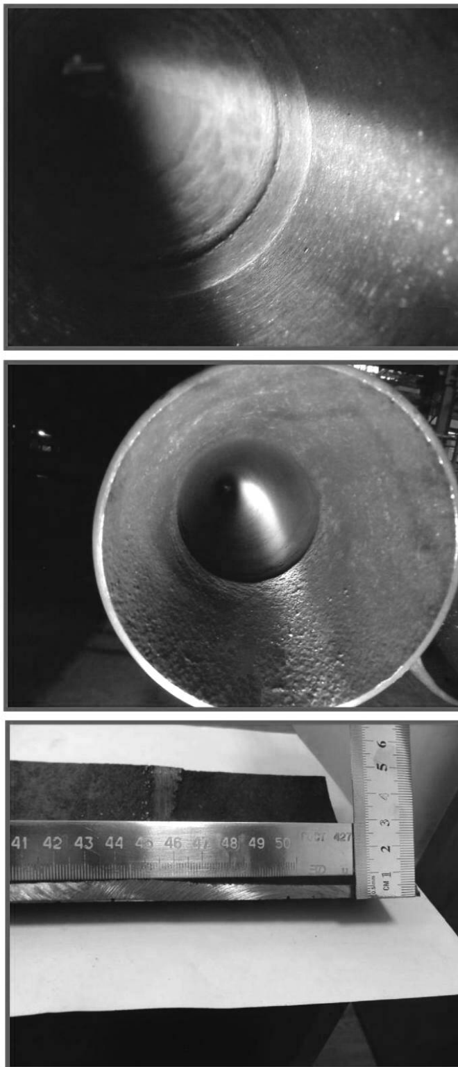
Рисунок Д.10 — Нарост, залив, грубая поверхность
