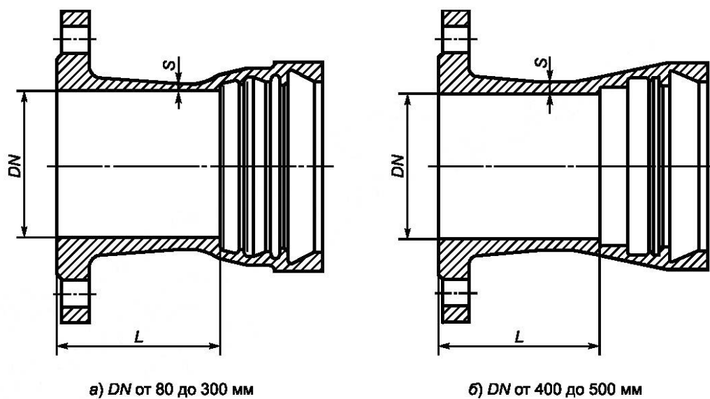
Рисунок Б.8 — Патрубок фланец — раструб (ПФР)
