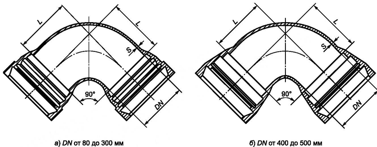
Рисунок Б.3 — Колено раструбное (УР)
