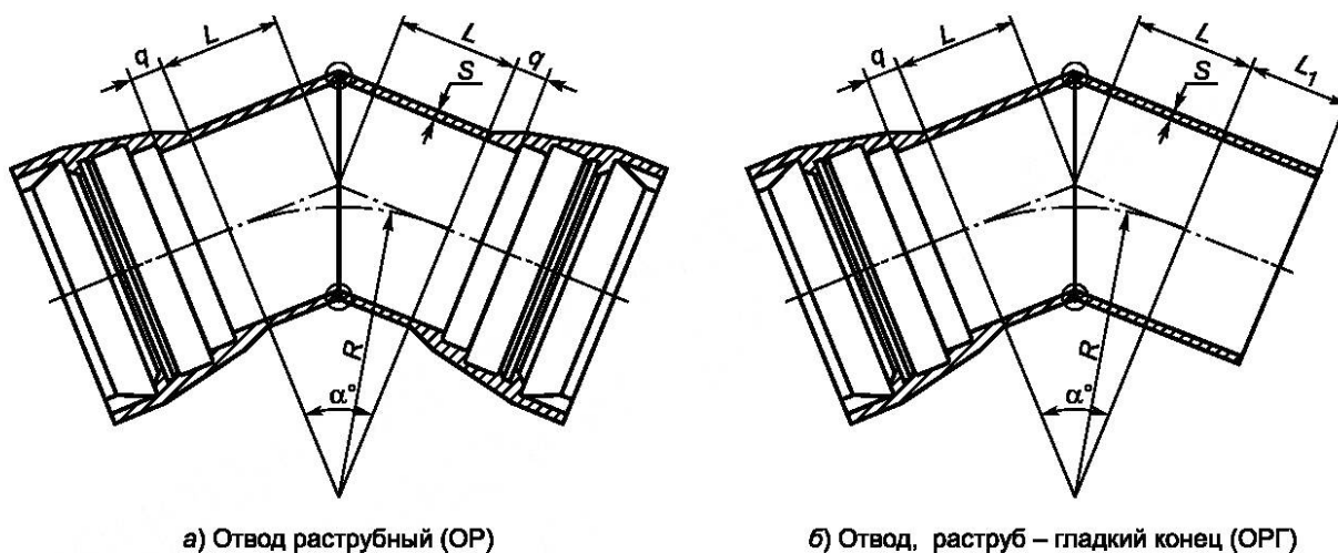
Рисунок В.5 — Отвод \alpha = 10^\circ/15^\circ/30^\circ (ОР, ОРГ)
