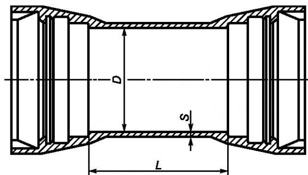
Рисунок Б.12 — Муфта надвижная (МН)
