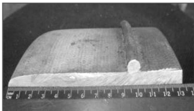
Рисунок Д.7 — Утонение гладкого конца трубы
