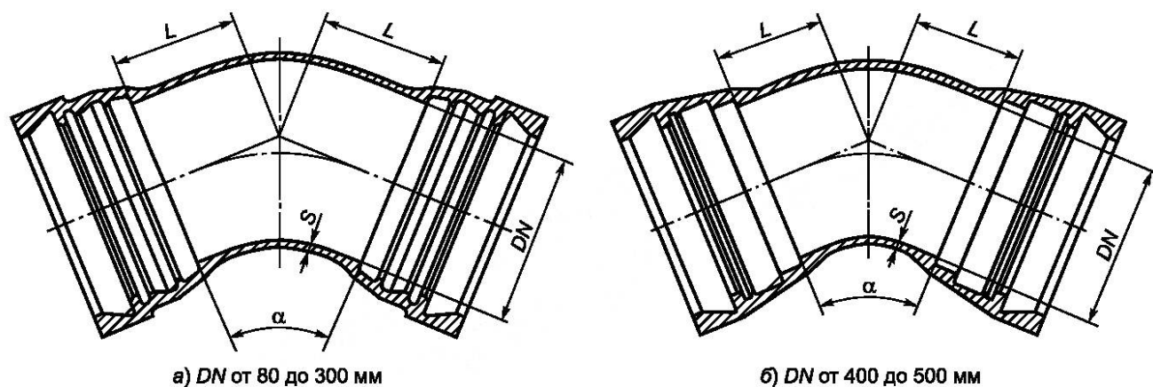
Рисунок Б.5 — Отвод раструбный (ОР)
