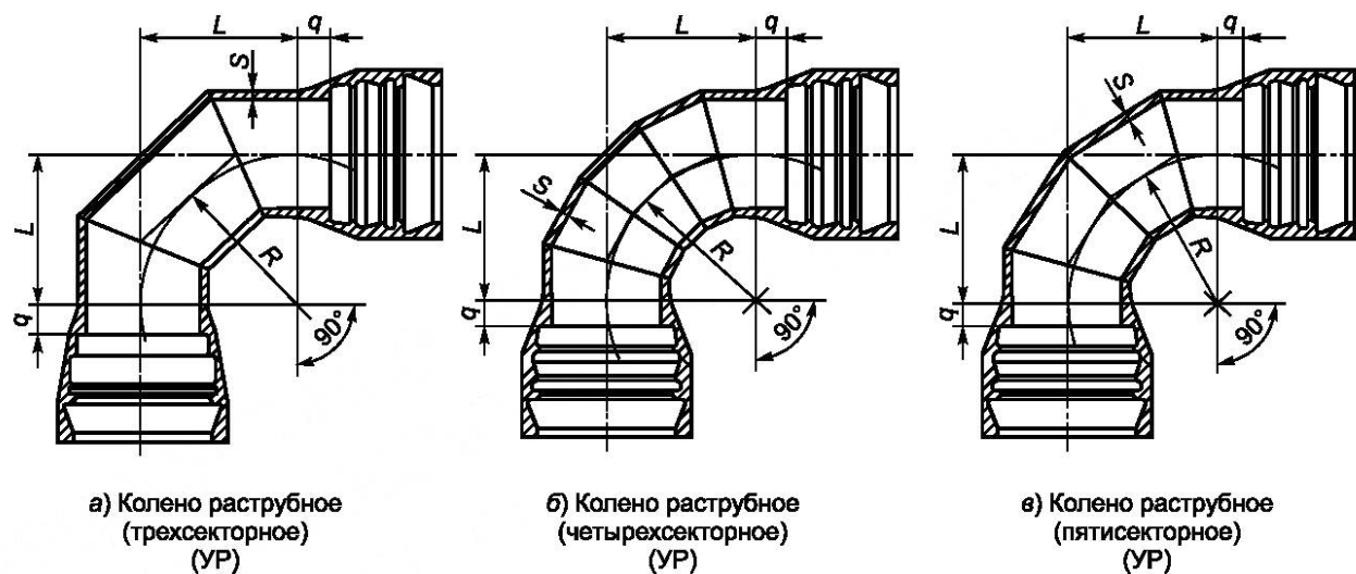
Рисунок В.4 — Колено (УР)
