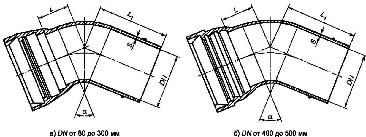
Рисунок Б.6 — Отвод, раструб — гладкий конец (ОРГ)
