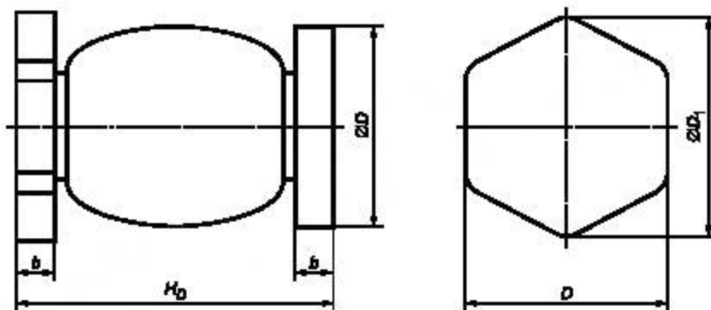
в) КД-35В
