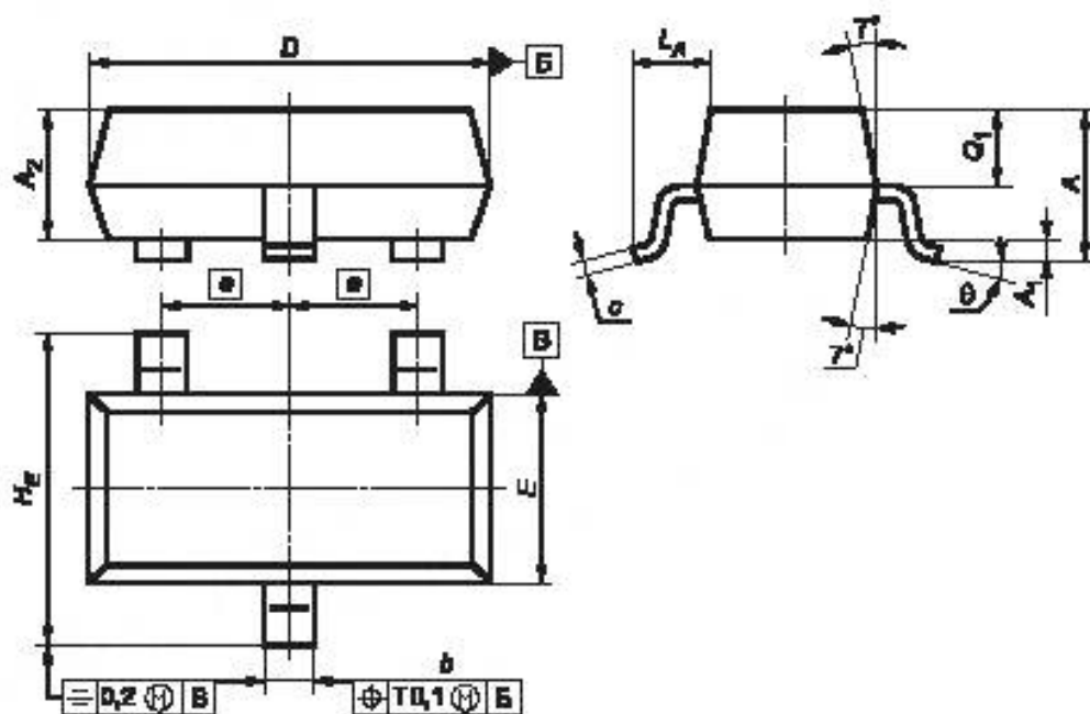
а) КТ-46
