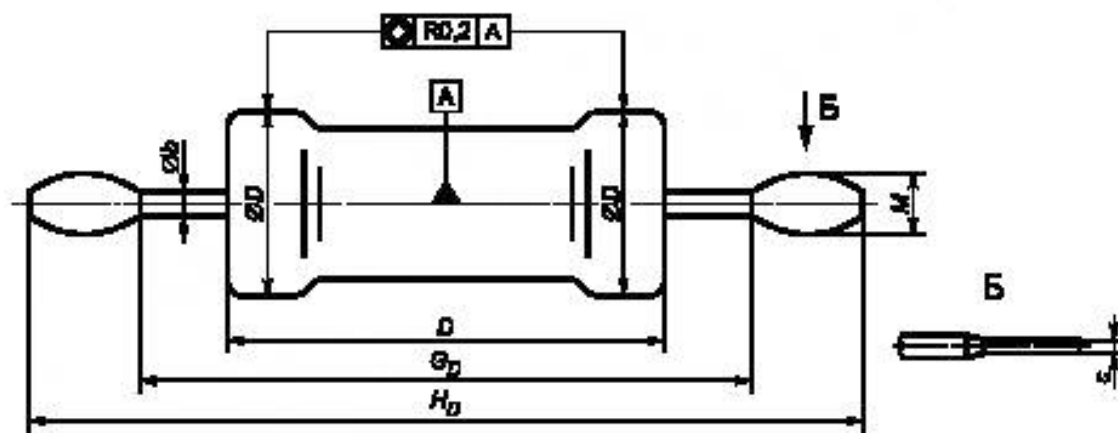
а) КД-121
