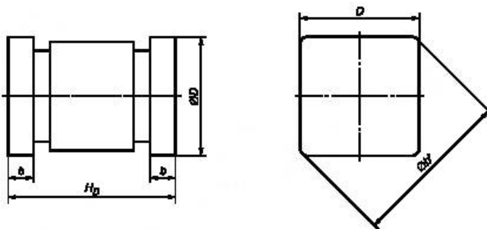
г) КД-35С
