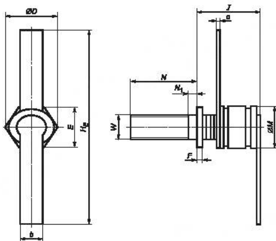
в) КД-10В
