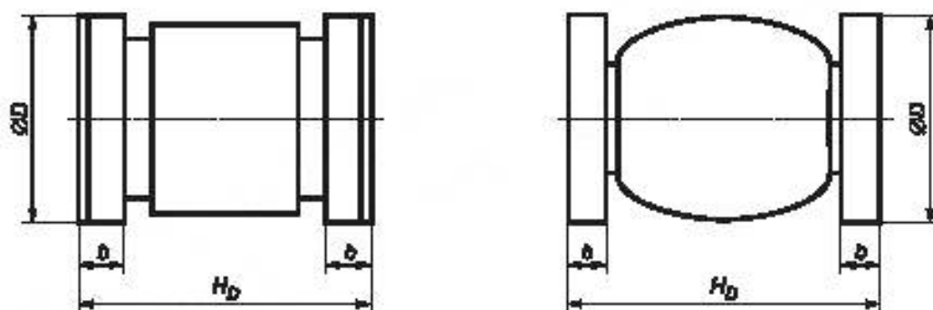
а) КД-35
