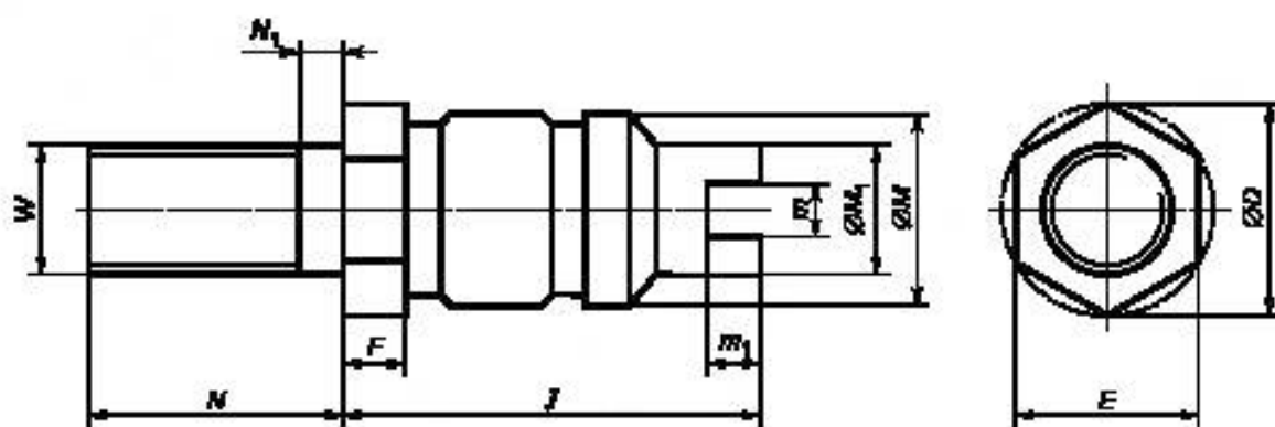
а) КД-10
