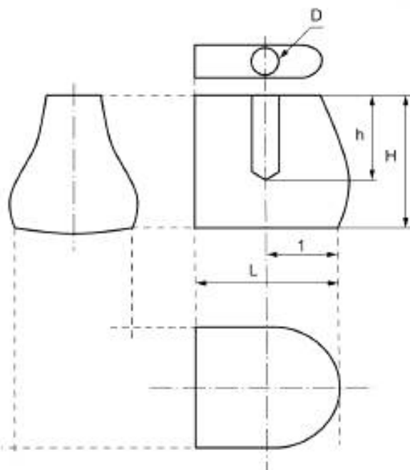
Рисунок 1 — Испытательное приспособление для определения энергии сжатия
