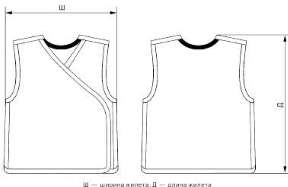
Рисунок 1 — Параметры защитного жилета
