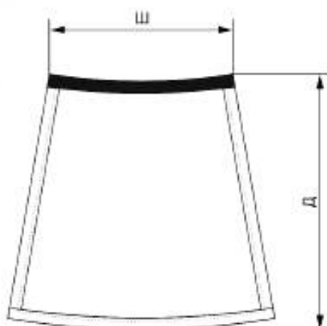
Рисунок 2 — Параметры защитной юбки
