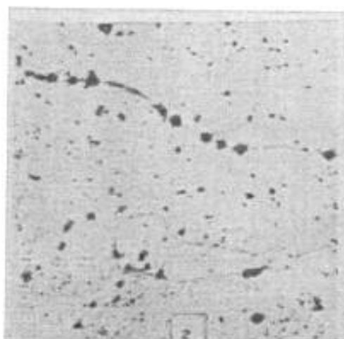
Растрав на поверхности штамповки в – макроструктура, г – микроструктура
