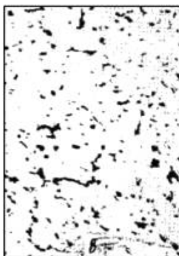
Микроструктура штамповки из сплава АК4-1. X250
