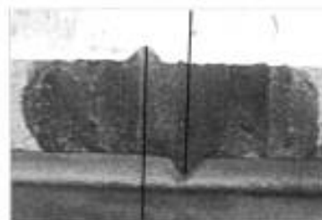
Риски на облое для контроля смещения
