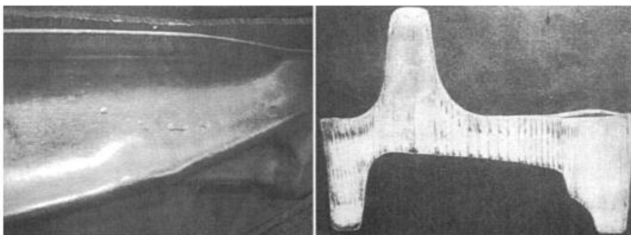
Рисунок А.22 — Пузыри
