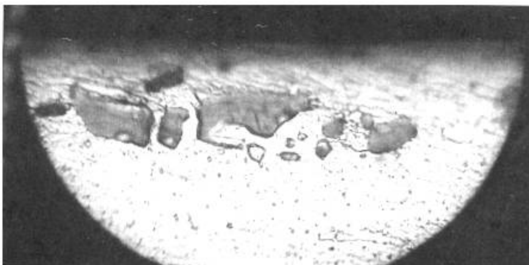
Микроструктура ликвационных скоплений в поверхностном слое штамповки. *100
