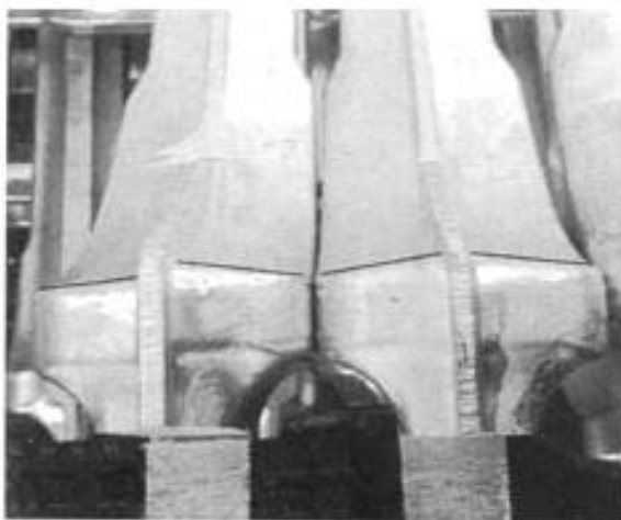
Смещение на штамповке
