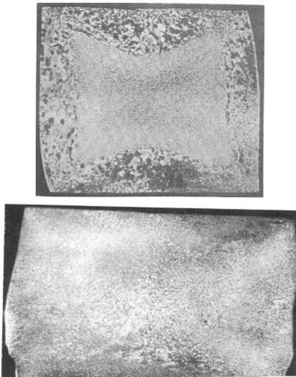
Макроструктура поковки
