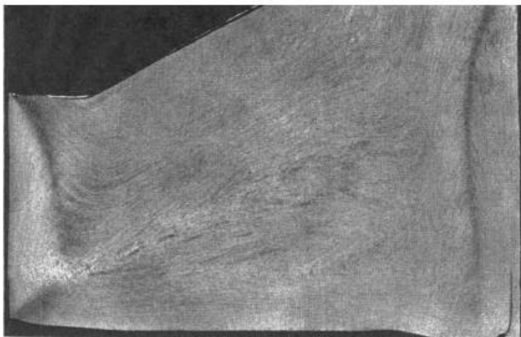
Рисунок А.12 — Утяжина
