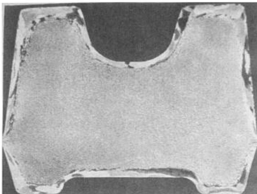
Рисунок А.3 — Крупнокристаллический ободок
