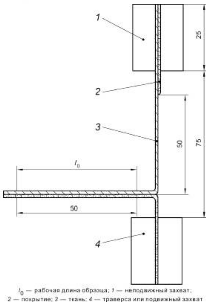
Рисунок Н.1 — Установка образцов тканей с толстыми покрытиями
