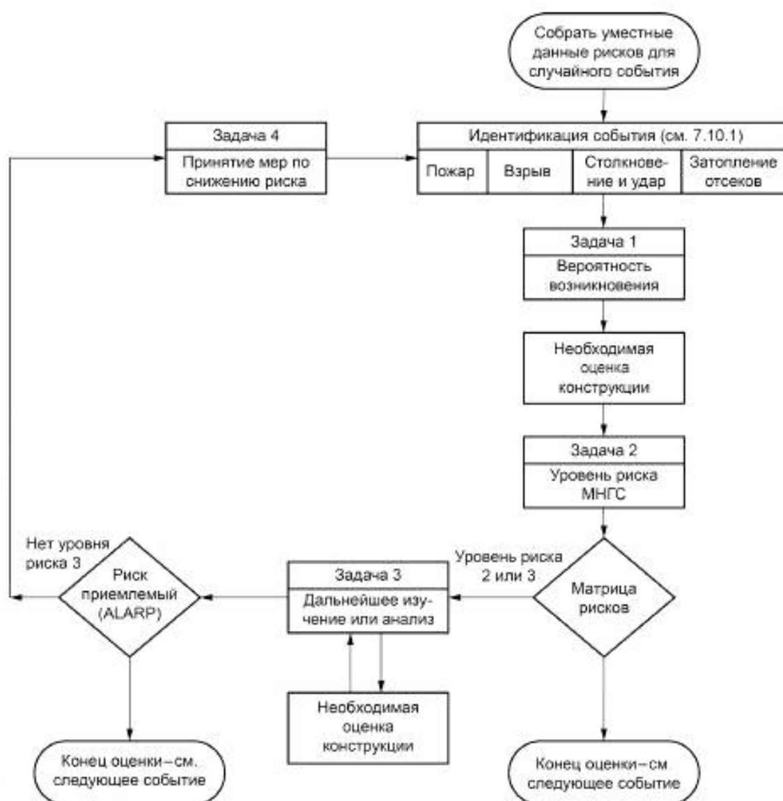
Рисунок 1 — Оценка аварийных ситуаций
