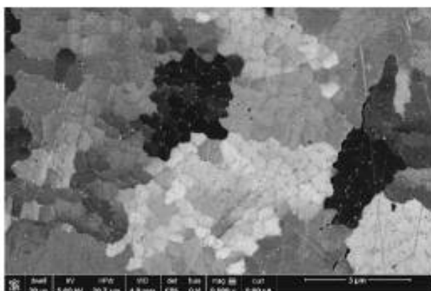
Рисунок 3 — Фронты кристаллизации (а) и ячейки (б) структуры образца
