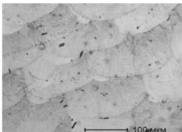
Рисунок 3 — Фронты кристаллизации (а) и ячейки (б) структуры образца
