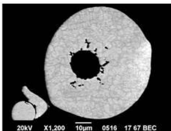
Рисунок 2 — Строение и морфология частиц: дендритное строение частицы (а), сателлиты (б) и аморфный панцирь (в) на поверхности частицы; пора (г)
