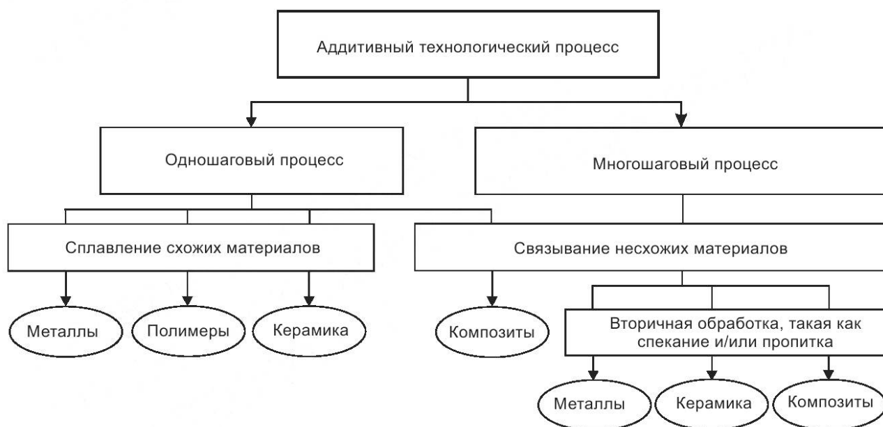
Рисунок В.1 — Принципы деления одношаговых и многошаговых аддитивных технологических процессов
