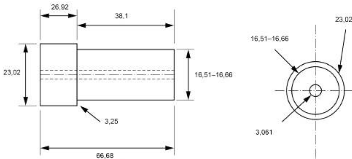
Рисунок 1 — Центрирующее устройство для центровки иглы
